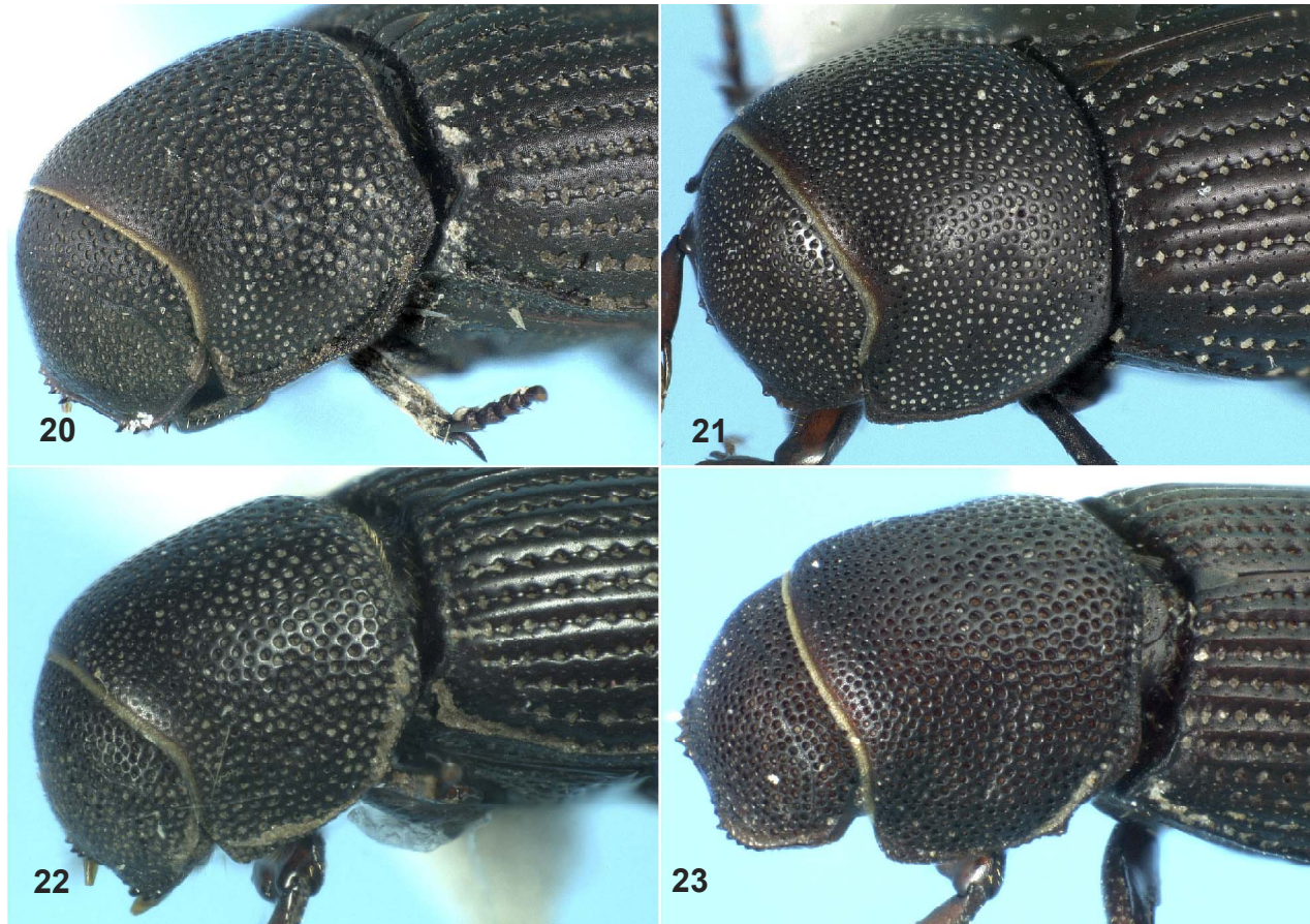
Figure 20-23. Saprostitellus spp., head to elytral bases. 20) Saprostitellus peruanus Stebnicka, holotype. 21) Saprostitellus kenodontus , n. sp. 22) Saprostitellus denticulatus Balthasar. 23) Saprostitellus ariquemus Stebnicka.
