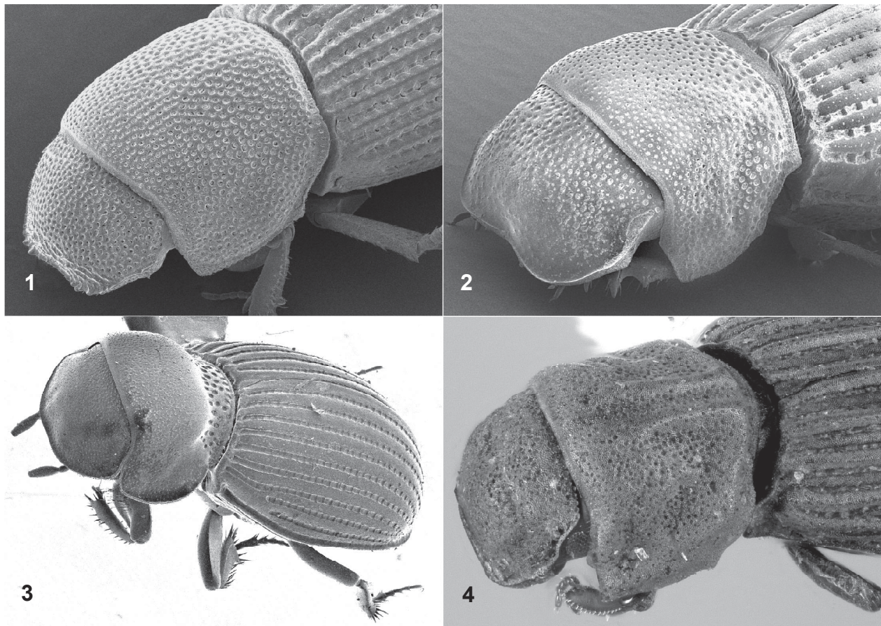
Figure 1-4. Key characters. 1) Saprositellus ariquemeres Stebnicka, head and pronotum. 2) Saprolochus tambopatae Stebnicka and Galante, head and pronotum. 3) Stebnickiella zosterixys , n. gen., n. sp., lateral habitus. 4) Amerilochus cinereus , n. gen., n. sp., head and pronotum.
