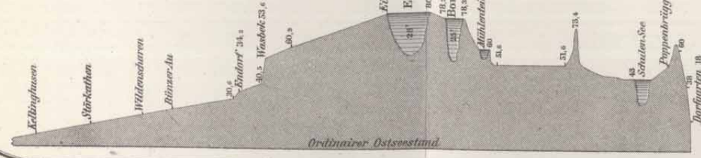
PROFIL ZWISCHEN DEM KIELER HAFEN UND DER STÖR.
