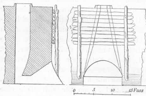
Fig. 28. 29. Eisenschmelzofen aus Birma. Nach BLANFORD.
