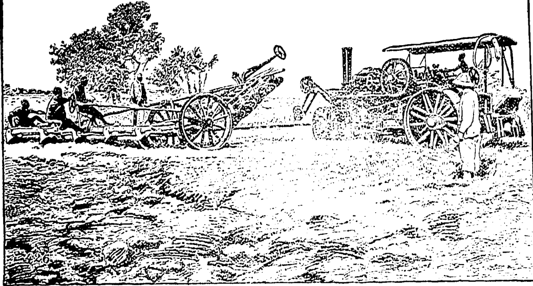
Kemnas Heißdampfplug auf einer Plantage in Kingwangwanda der Deutschen Rufiji Baumwoll-Gesellschaft in Tätigkeit.
