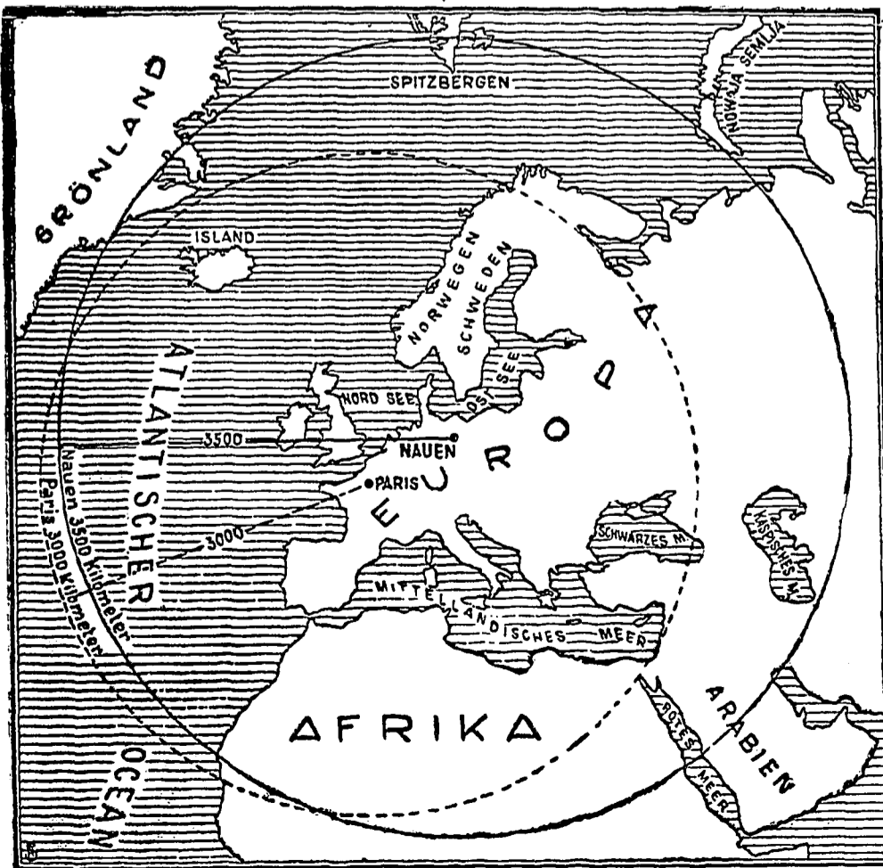
Die normale Reichweite der Stationen für Funkentelegraphie Nauen und Paris.
