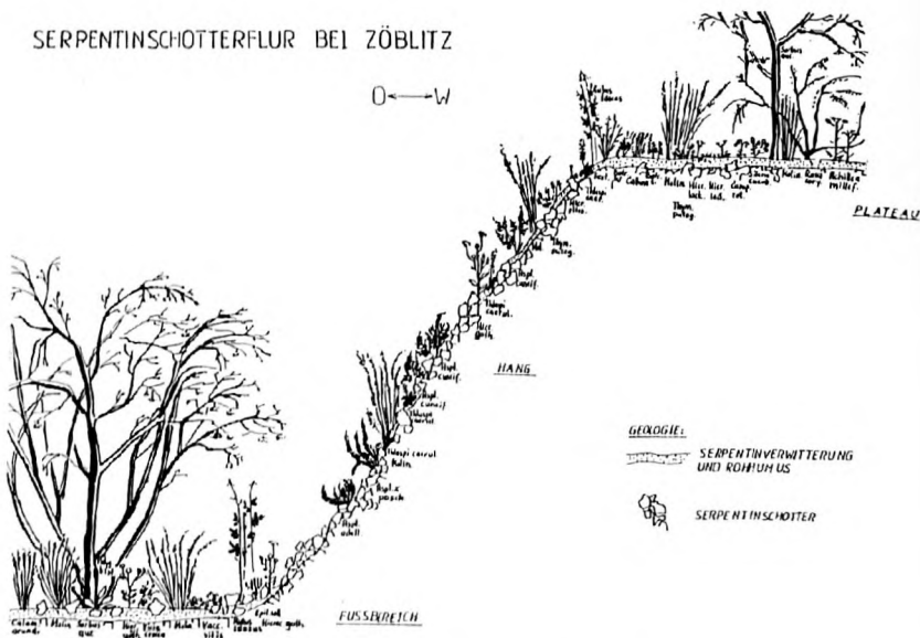
Abb. 1: Übersicht des erfaßten Transektes mit den drei Abschnitten Plateau, Hang und Hangfuß.
