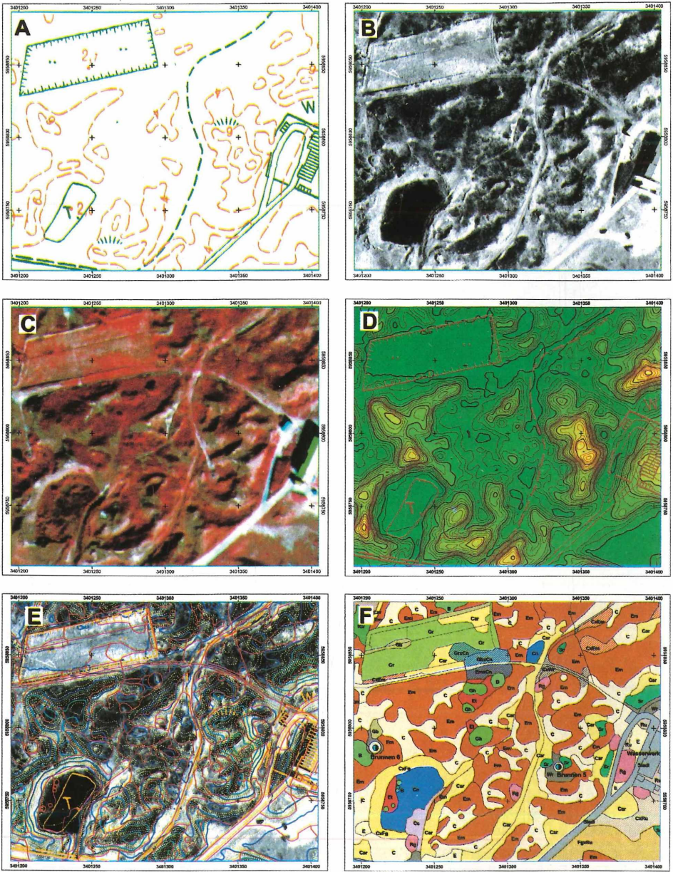
Abb. 27: Datengrundlage und Ergebnisse der Vegetationskartierung am Beispiel eines Detail-Bereiches vom Grundwasser-Einzugsgebiet der Insel Langeoog (A: Deutsche Grundkarte, B: Schwarz-Weiß-Luftbild, C: Color-Infrarot-Luftbild, D: Höhenmodell, E: Feldkarte und F: Vegetationskarte, nach PETERSEN et al. 2003).
