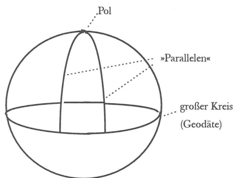
Abb. 2: Veranschaulichung von Riemanns sphärischer Geometrie
