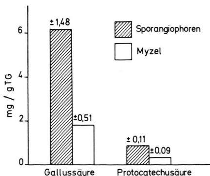
Abb. 3. Gallus- und Protocatechusäurekonzentration von Sporangiphoren und Myzel einer 5 Tage alten Dunkelkultur mit Zinkzusatz.
