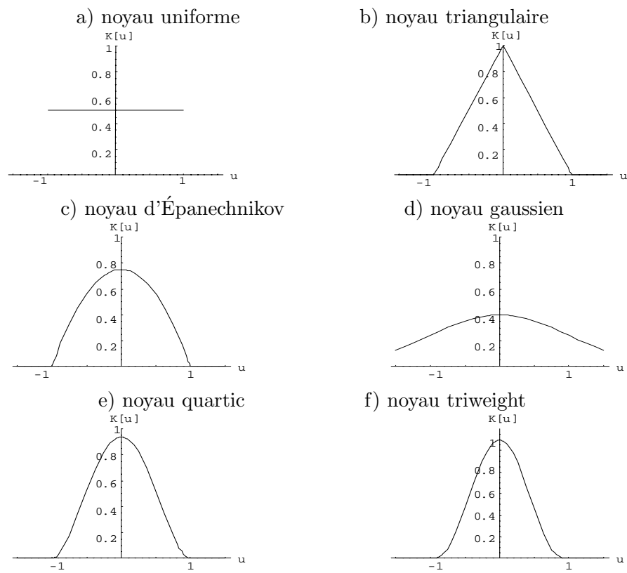
Graphique 2 – Représentations graphiques des noyaux
