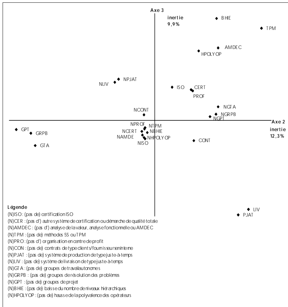
Graphique 3 – Représentation dans le plan engendré par les deuxième et troisième axes factoriels de l'ACM réalisée à partir des treize dispositifs.
