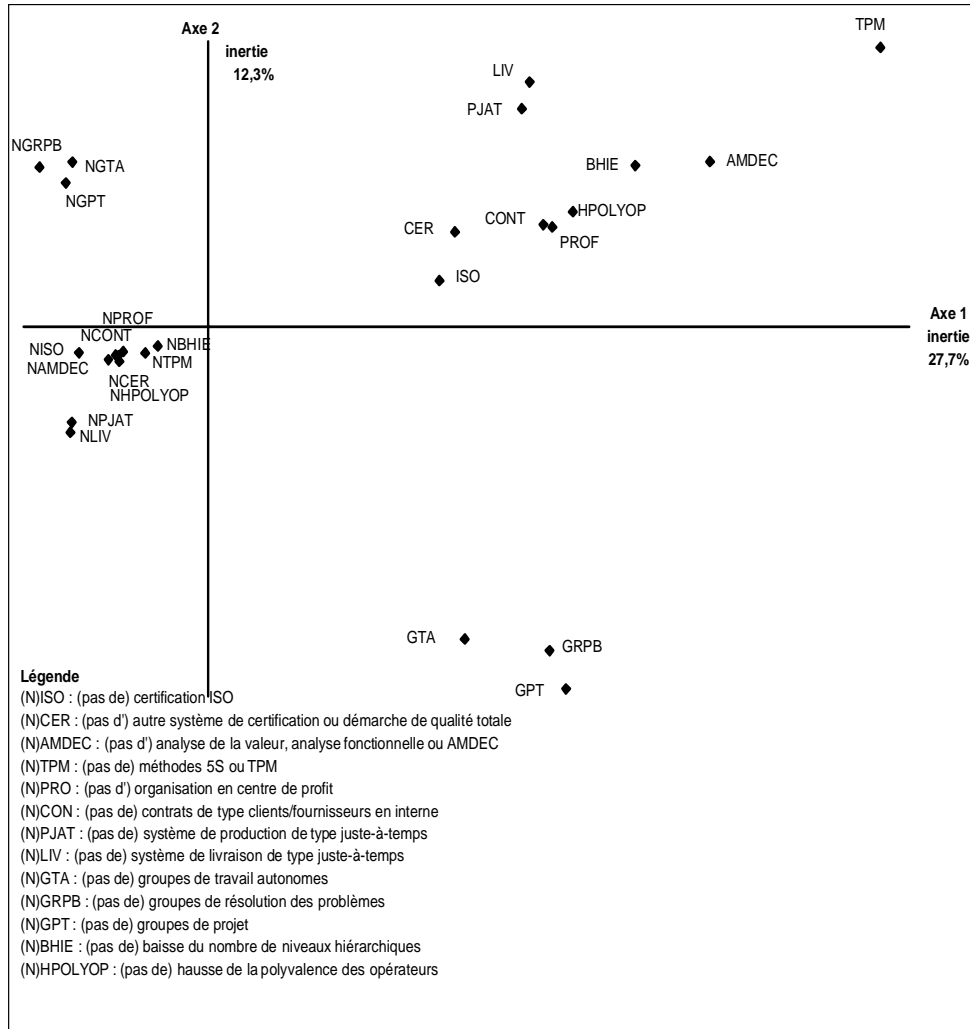
Graphique 2 – Représentation dans le plan engendré par les deux premiers axes factoriels de l'ACM réalisée à partir des treize dispositifs
