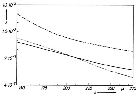
Abb. 2. Der Absorptionskoeffizient von einigen Quarzgläsern: Herasil I (—), Suprasil (---) und Infrasil (·····).
