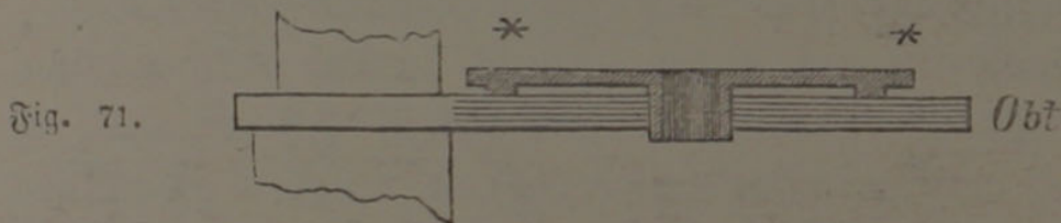
Fig. 70. Federklammer im Durchschnitte gesehen. Fig. 71. Welcker's drehbarer Objecttisch im Durchschnitte.
