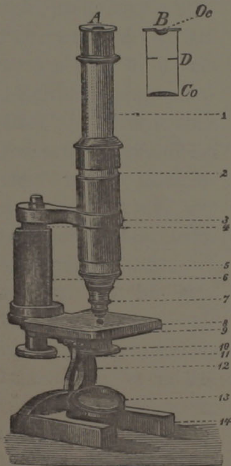
Fig. 33. A Mikroskop aus der Werkstätte von N. Winkel in Göttingen.
