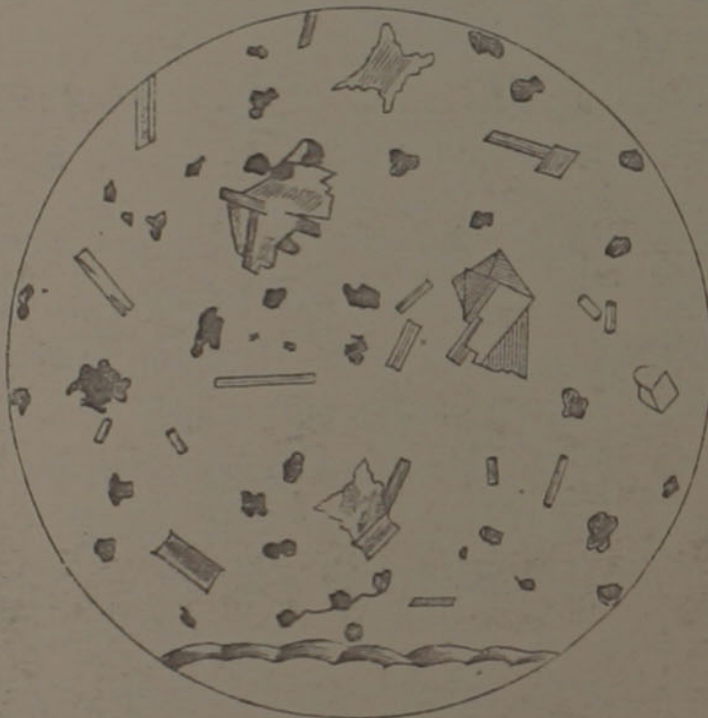
Fig. 123. Obsidian aus Mexico. Dünnschliff.
