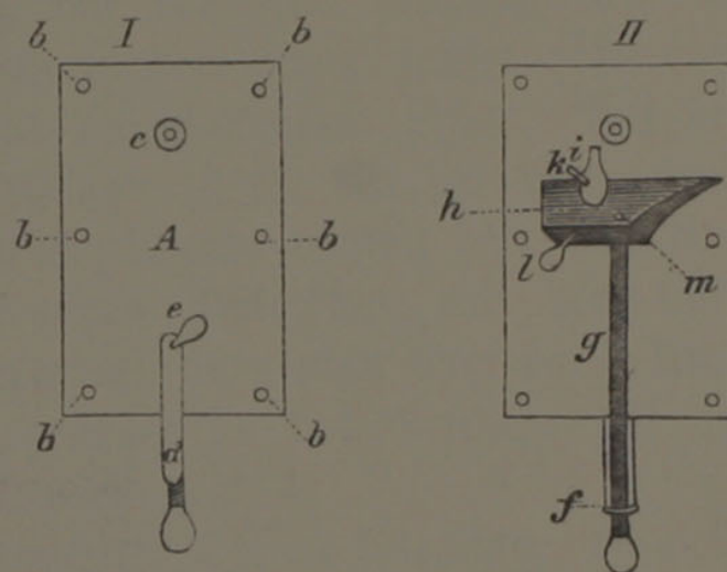
Fig. 44. Leeuwenhoek's Mikroskop.
