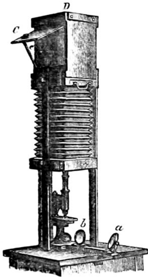
Fig. 82. Photographischer Apparat. (Nach Robin.)
