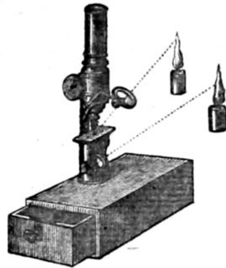
Fig. 54. Zusammengesetztes Mikroskop von Fraunhofer. (Nach Chevalier.)
