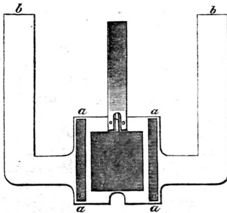
Fig. 74. Heizbarer Objecttisch von M. Schulze.
