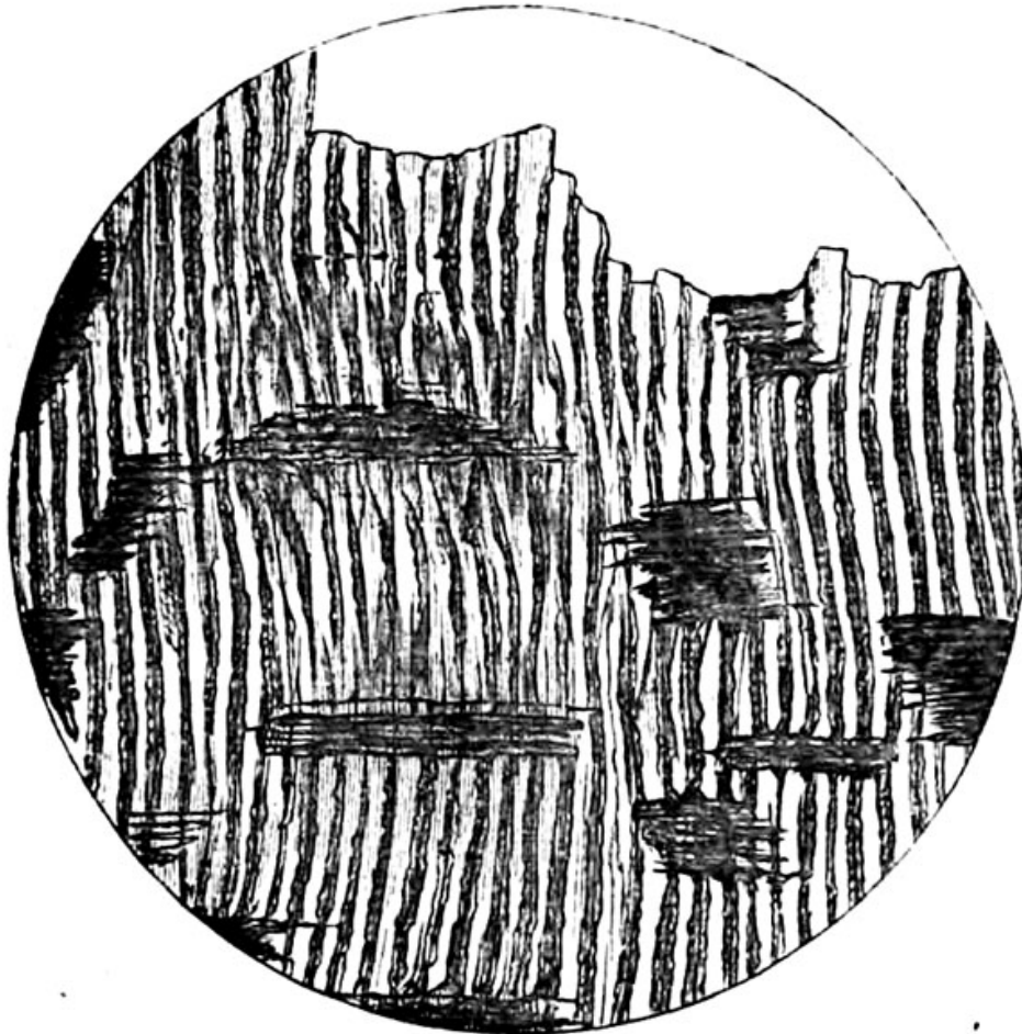
Fig. 125. Steinkohle, Dünnschliff.
