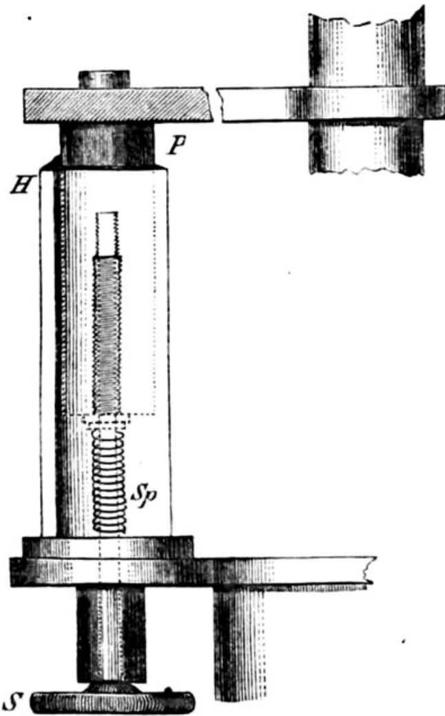
Fig. 34. Mikrometerschraube in schematischer Zeichnung
