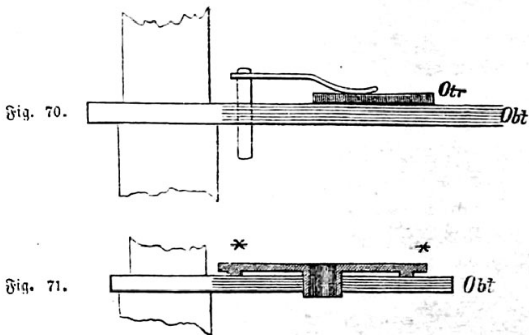
Fig. 70. Federklammer im Durchschnitte gesehen. Fig. 71. Welcker's drehbarer Objectisch im Durchschnitte.
