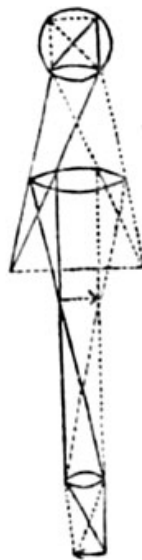
Fig. 40. Griendel von Ach's Mikroskop. (Nach der Originalabbildung.)
