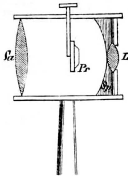
Fig. 48. Lieberkühn'sches einfaches Mikroskop.
