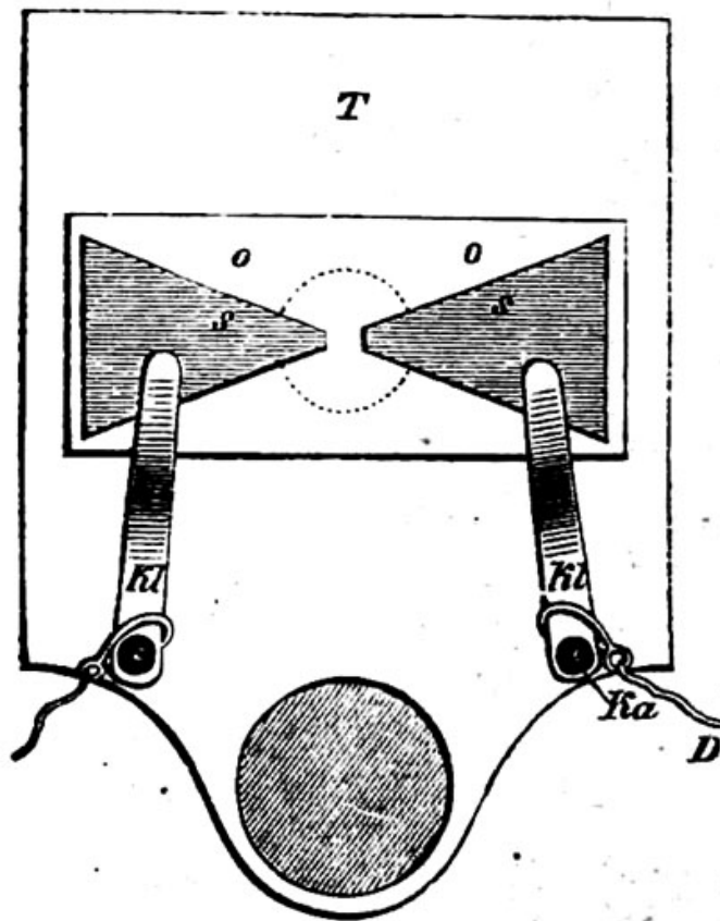
Fig. 73. Electrischer Objectträger.
