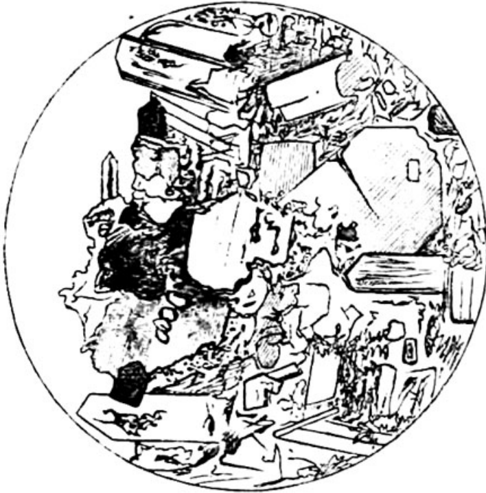
Fig. 122. Lava vom Vesuv. Dünnschliff.
