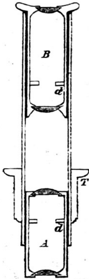
Fig. 65. Hartnack's bildumkehrendes Ocular. A Doublett. B Ocular. T Tubus des Mikroskopes. dd Diaphragmen.
