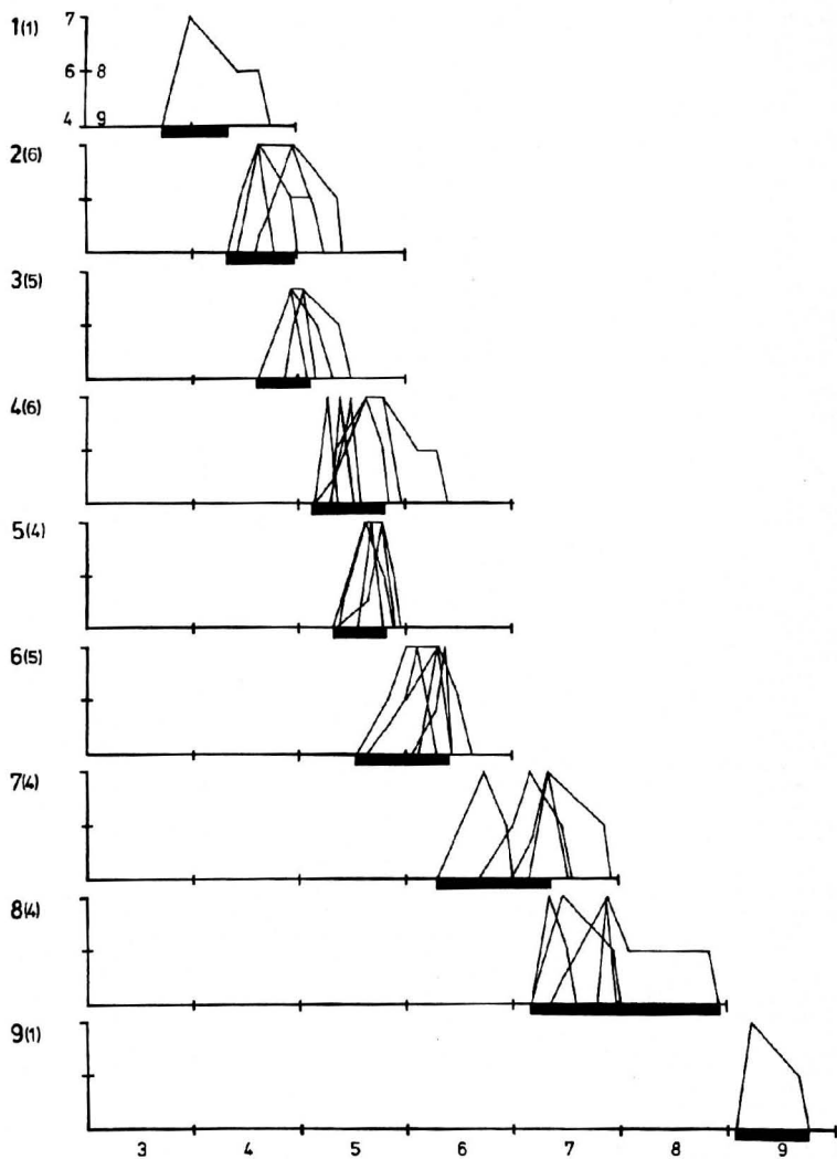
Abb. 2: Blühwellen der Krautschicht von Buchenwäldern ( Melico-Fagetum ) in der Umgebung von Göttingen (nach Beobachtung von 4 Flächen 1971).
