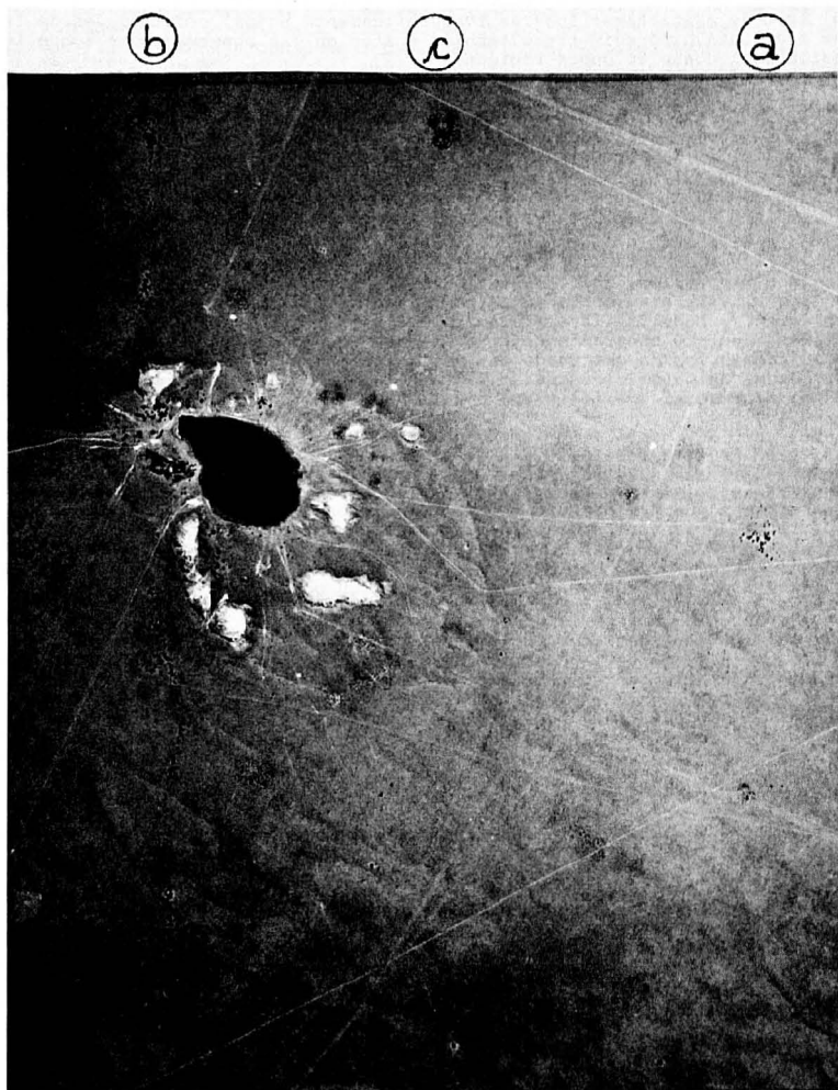
Figura 3: Fotografía aérea del pastizal de psamófitas. Laguna Las Vacas al SW de Villa Mercedes.
