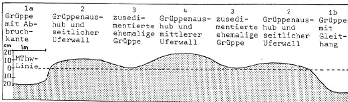
Abb. 3: Schematisches Querprofil durch ein Gruppenbeet mit dem Mikrorelief und den unterschiedlichen Kleinstandorten (s. dazu auch die Profile mit den Pflanzengesellschaften, Abb. 11).
