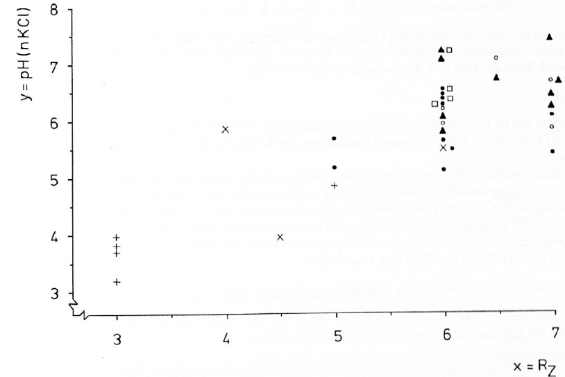
Abb. 2: Beziehungen zwischen den zentralen Reaktionszahlen ( R_z ) und den pH(n KCl)-Werten in holsteinischen Erlenwäldern nach Daten von MÖLLER (1970). (Die pH-Werte gelten für die oberen 30 cm des Torf- bzw. Anmoorkörpers. Näheres s. Text.)
