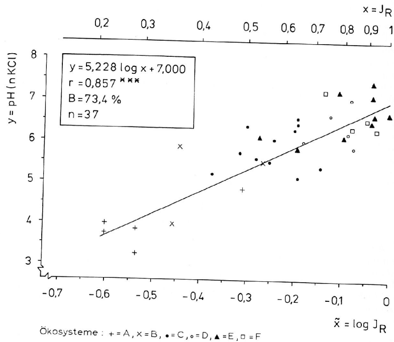
Abb. 3: Beziehungen zwischen den Logarithmen der Reaktionszahlen-Indices ( \log I_R ) und den \text{pH}(\text{nKCl}) -Werten in holsteinischen Erlenwäldern nach Daten von MÖLLER (1970). (Die \text{pH} -Werte gelten für die oberen 30 cm des Torf- bzw. Anmoorkörpers. Näheres s. Text.)
