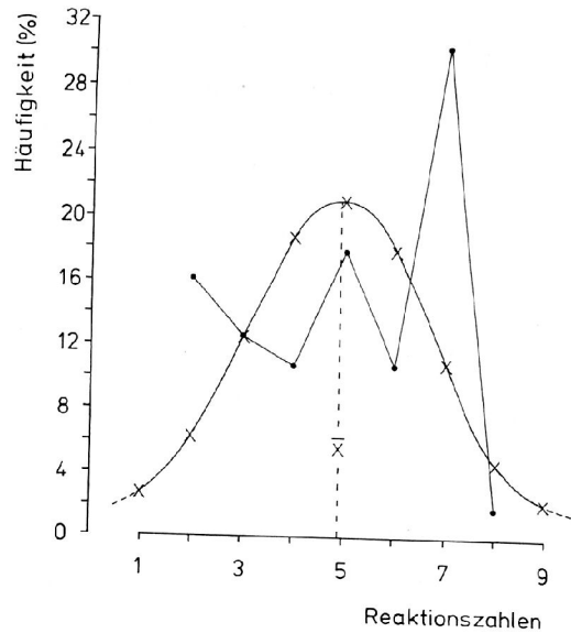
Abb. 1: Vergleich von theoretischer Normalverteilung ( x-x ) und tatsächlich vorgefundener Verteilung ( \bullet-\bullet ) der Reaktionszahlen am Beispiel der Aufnahmen 44 bis 48 aus Vegetationstabelle 1 ( Carici elongatae-Alnetum glutinosae , trennartenfreie Subassoziation) von MÖLLER (1970) ( \bar{x} \pm s = 4,93 \pm 1,90 ).
