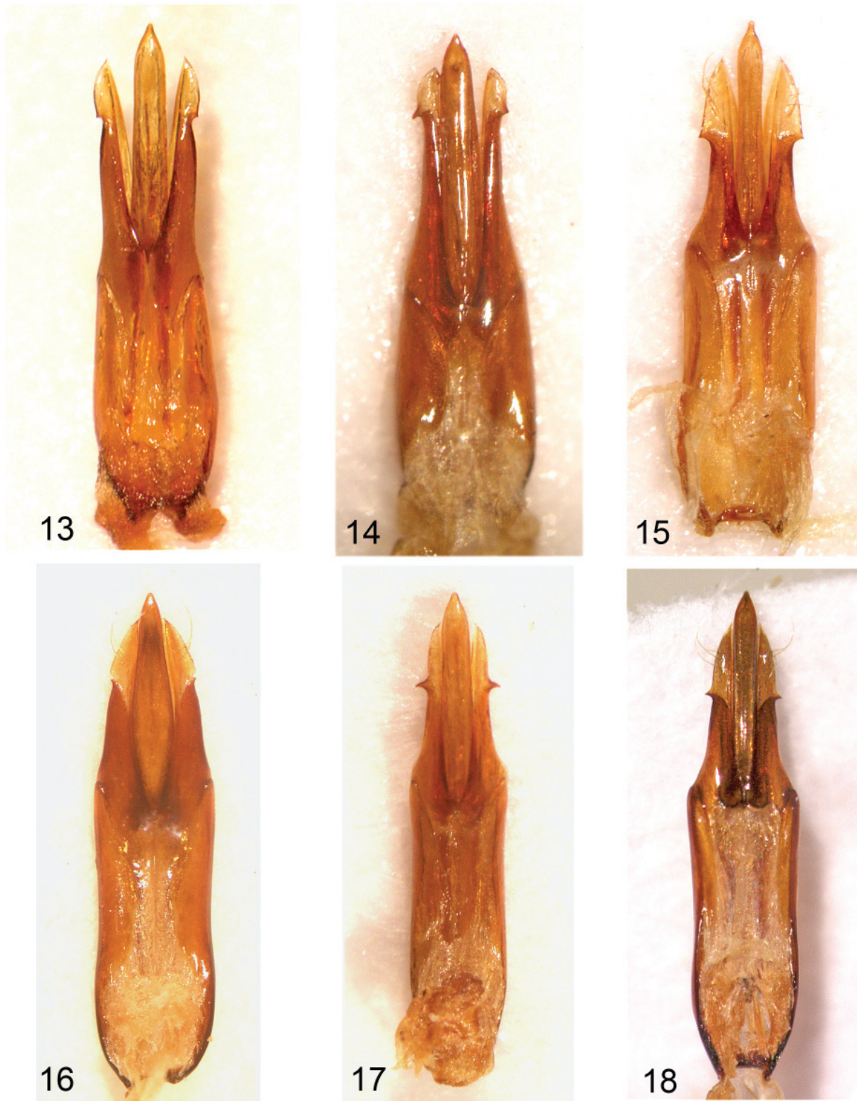
Figures 13-18. Dipropus species, aedeagi, dorsal aspects. 13) D. pericu n. sp. 14) D. reinae n. sp. 15) D. sonora n. sp. 16) D. sus (Candèze). 17) D. warneri n. sp. 18) D. yaqui n. sp.
