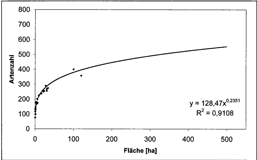
Abb. 1: Zusammenhang zwischen Flächengröße und Artenzahl für 26 Bahnhöfe in Deutschland.
