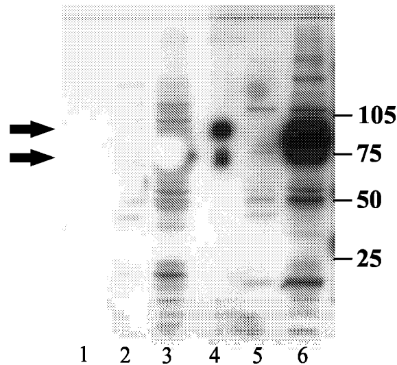
Abb. 3.20. Westernblotanalysen unter Verwendung des EnvB2-2 Serums.
