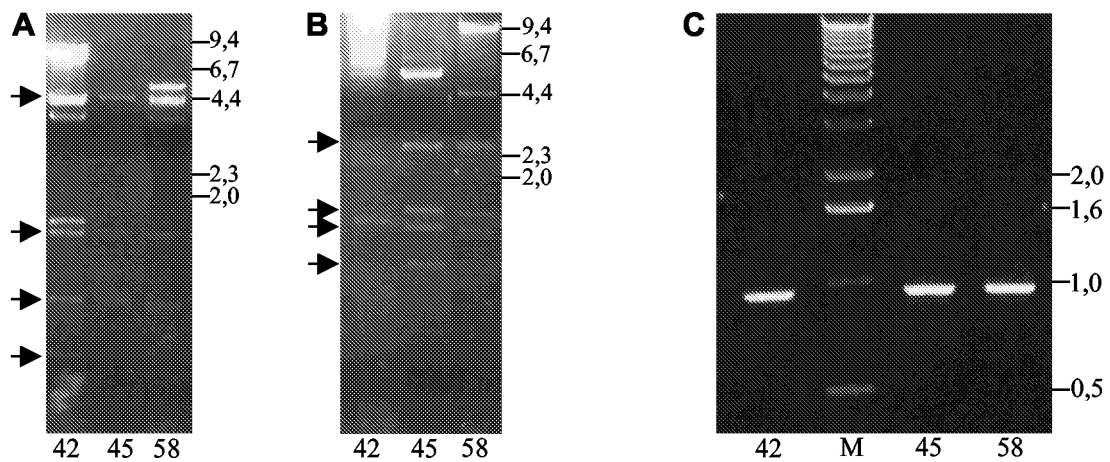
Abb. 3.25. Restriktionsanalyse und Integrationsnachweis der PK15-PERV-A Klone.
