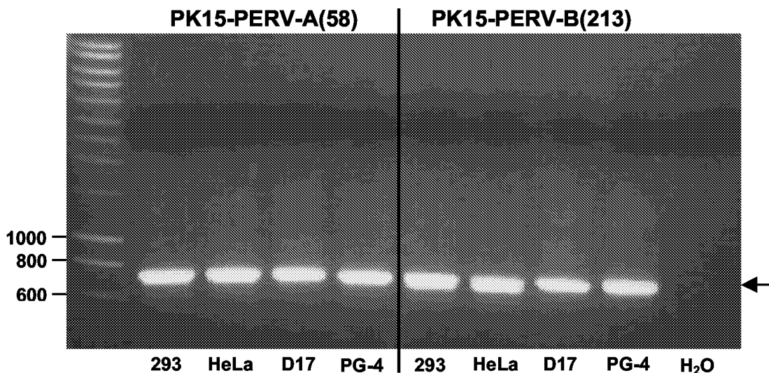
Abb. 3.34. Integrationsnachweis der viralen DNA nach Infektion mit PK15-PERV-A(58) und PK15-PERV-B(213).
