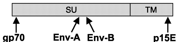
Abb. 3.15. Schematische Darstellung der Lokalisation der Peptide gerichtet gegen PERV Env.
