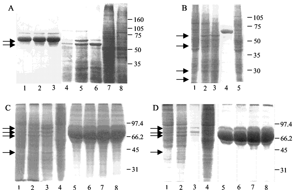
Abb. 3.1. SDS-PAGE mit Zellysaten von PERV-Protein exprimierenden Insektenzellen.
