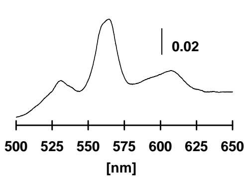
Abb. 26: Natives Redox-Spektrum der Cyto Chinoloxidase aus dem P. denitrificans -Stamm ORI2K31. Das Dithionit-reduzierte minus oxidierte Differenzspektrum wurde bei einer Proteinkonzentration von 0,18 mg/ml aufgenommen.
