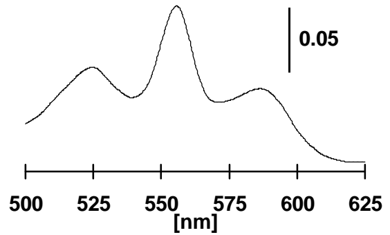
Abb. 27: Pyridin-Hämochrom-Spektrum der Cyto Chinoloxidase aus dem P. denitrificans -Stamm ORI2K31. Das Spektrum wurde bei einer Proteinkonzentration von 0,4 mg/ml aufgenommen.
