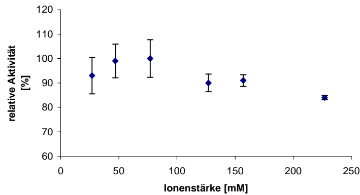
Abb. 22: Relative Aktivität der ba 3 Chinoloxidase in Abhängigkeit von der Ionenstärke. Gemessen wurde in einem Puffer mit 10 mM KPi pH 7,4, 0,015% DM mit variabler KCl-Konzentration.
