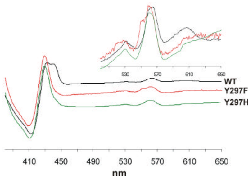
Abb. 32: Redox-Spektren der gereinigten ba 3 Chinoloxidasen. WT in schwarz, Y297F-Mutante in rot und Y297H-Mutante in grün. Spektren wurden auf gleiche Absorption im Soret-Bereich normiert.
