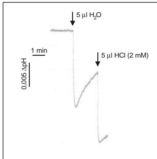
Abb. 31: Exemplarisches Schreiberprotokoll eines Protonen-Ganzzellpump-Experiments. Durch Pfeile sind die Zeitpunkte der Zugabe des Substrats (5 µl Sauerstoff-gesättigtes Wasser) sowie des Eichpulses (5 µl einer 2 mM HCl-Lösung) angegeben.
