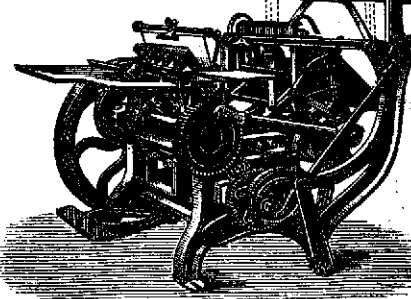
Liberty-Press mit Selbstausleger. Presse Liberty à levreur automatique. Liberty Press with automatic throw-off.
