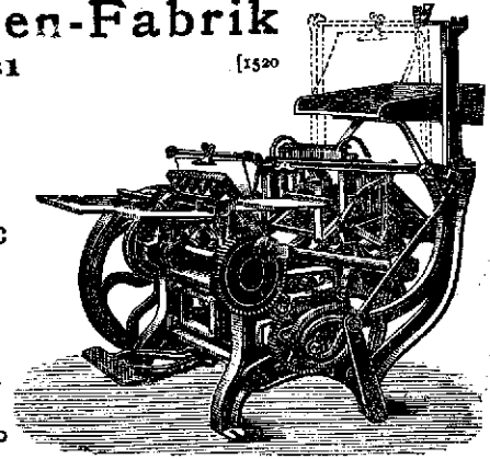
Liberty-Press mit Selbstausleger. Presse Liberty à levreur automatique. Liberty Press with automatic throw-off.
