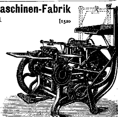
Liberty-Press mit Selbstausleger. Presse Liberty à leveur automatique. Liberty Press with automatic throw-off.
