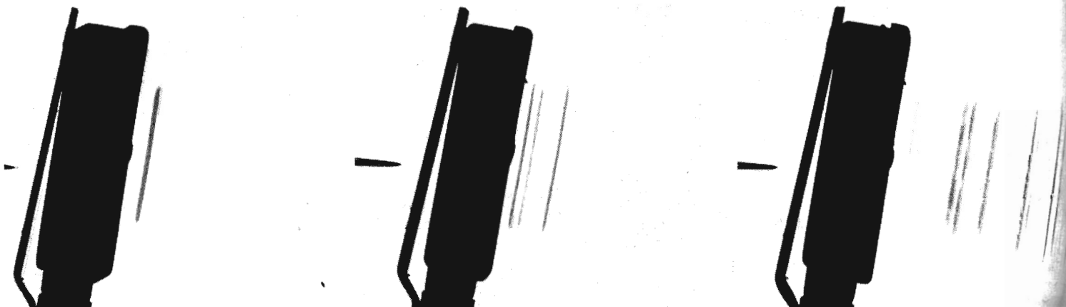
Bild 2: Sichtbarmachung von Ultraschallwellen. Die Aufnahmen zeigen die Ablösung von Ultraschallwellen von einem Schallsender, der sich unter Wasser befindet. Sie wurden mit Hilfe der Schlierenmethode sichtbar gemacht. Der zeitliche Abstand der einzelnen Bildphasen betrug \frac{1}{500.000} Sekunde; im üblichen Sprachgebrauch entspricht das einer Aufnahmefrequenz von 500.000 B/sec.
