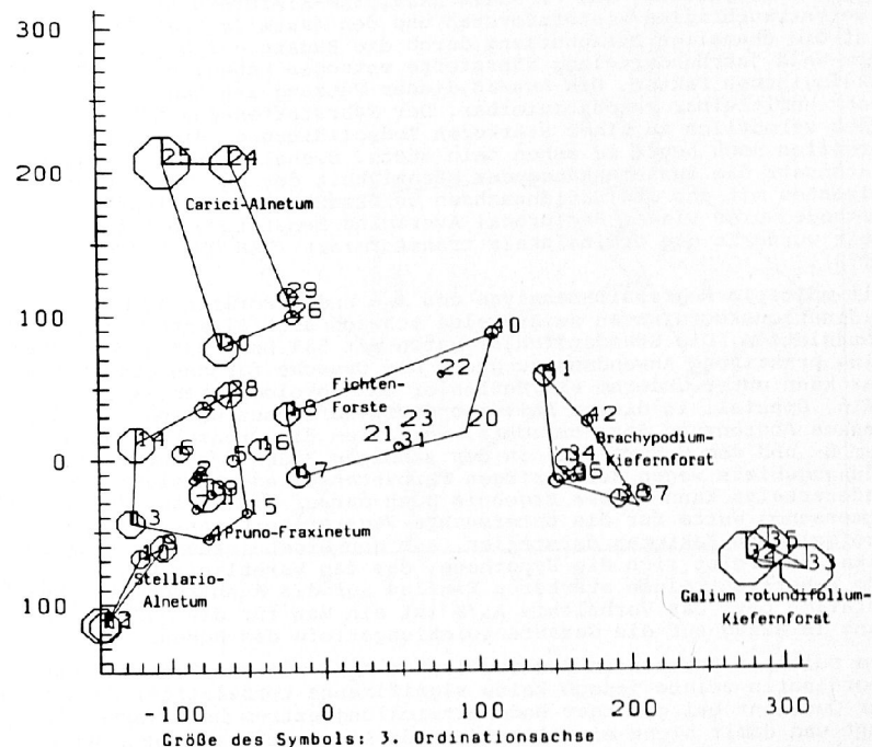
Abb. 1: Ordinationsdiagramm der Auwälder und Forste.
