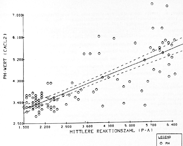
Abb. 4: Korrelation zwischen Reaktionszahl und pH-Wert.
