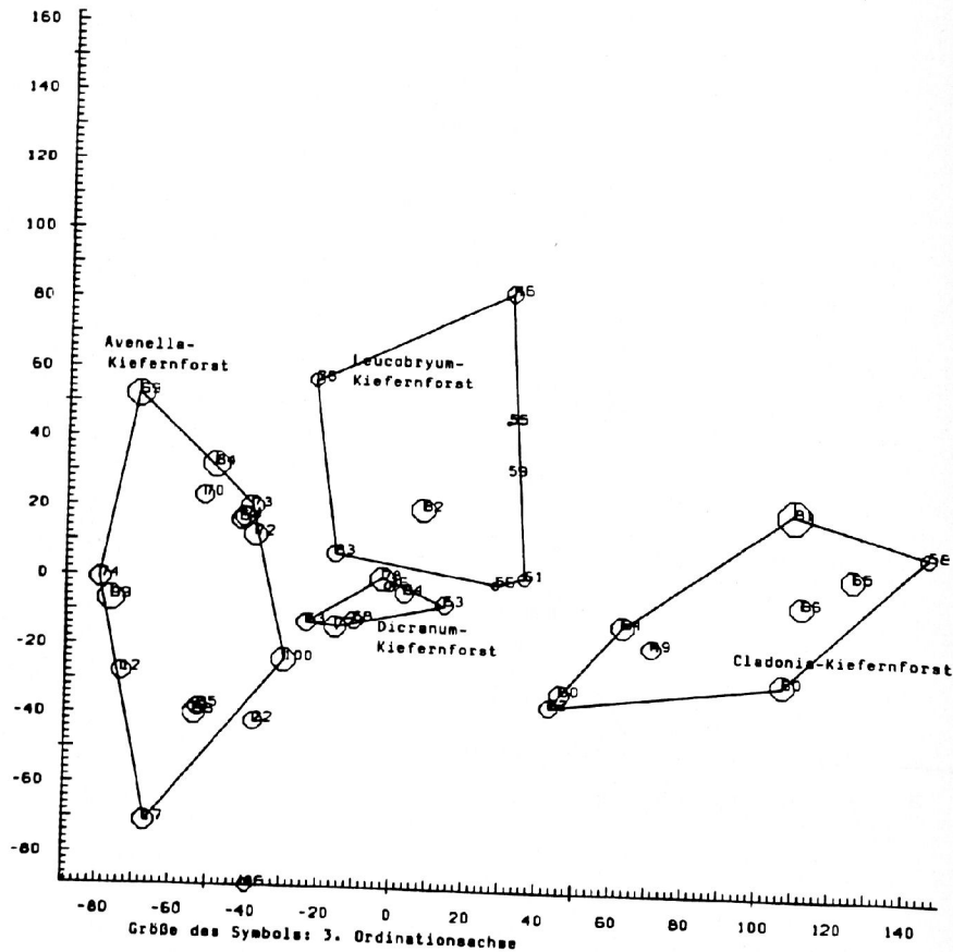
Abb. 3: Ordinationsdiagramm trockener Kiefernforste.
