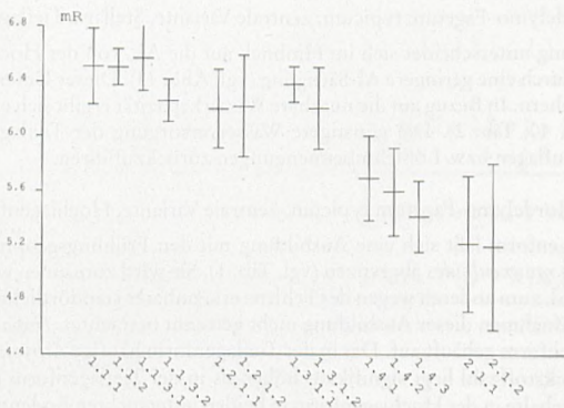
Abb. 18: Mittlere Reaktionszahl n. ELLENBERG für die verschiedenen Vegetationseinheiten (Mittelwert und Streuung).
