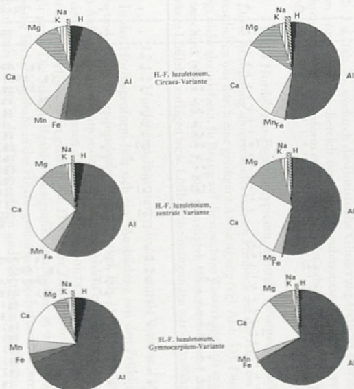
Abb. 14: Kationen-Sättigungsgrade der verschiedenen Ausbildungen des Hordelymo-Fagetum luzuletosum in zwei Bodentiefen (links: 0-8 cm, rechts: 8-15 cm).
