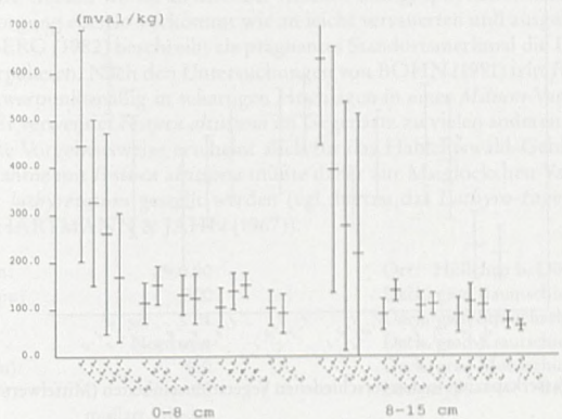
Abb. 7: effektive Austauschkapazität der verschiedenen Vegetationseinheiten in zwei Bodentiefen (Mittelwert und Streuung).
