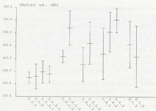
Abb. 3: Höhenlage der verschiedenen Vegetationseinheiten (Mittelwert und Streuung).
