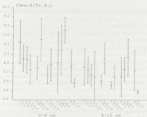
Abb. 19: Gehalte an organisch gebundenem Kohlenstoff in den verschiedenen Vegetationseinheiten in zwei Bodentiefen (Mittelwert und Streuung).
