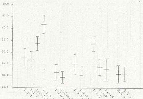
Abb. 9: Artenzahlen der verschiedenen Vegetationseinheiten (Mittelwert und Streuung).
