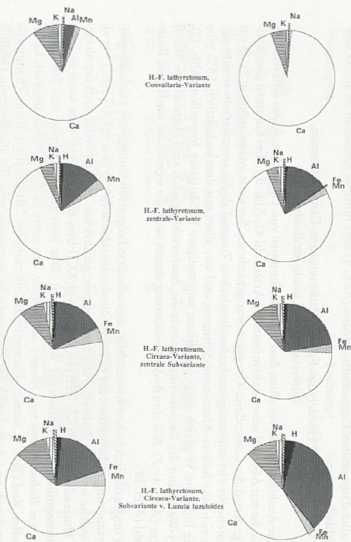
Abb. 12: Kationen-Sättigungsgrade der verschiedenen Ausbildungen des Hordelymo-Fagetum lathyretosum in zwei Bodentiefen (links: 0-8 cm, rechts: 8-15 cm).
