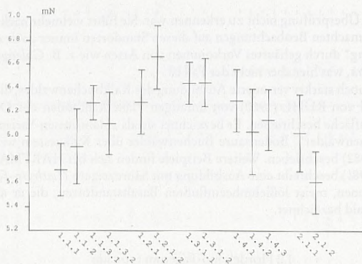
Abb. 16: Mittlere Stickstoffzahl n. ELLENBERG für die verschiedenen Vegetationseinheiten (Mittelwert und Streuung).
