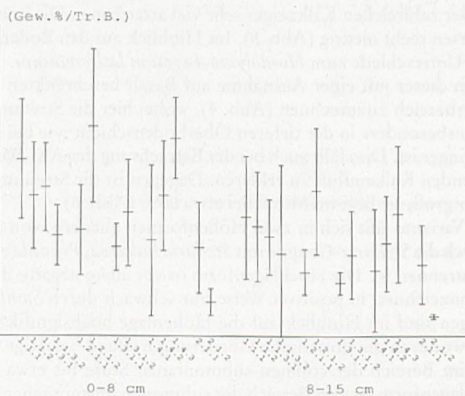
Abb. 17: Gesamt-Stickstoffgehalte der verschiedenen Vegetationseinheiten in zwei Bodentiefen (Mittelwert und Streuung).
