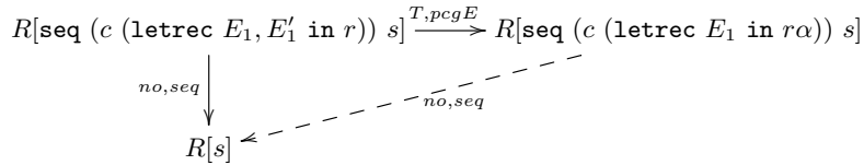
(d) Typical case for diagram (9)
