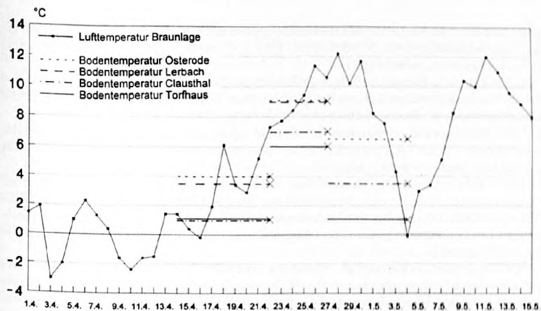
Abb. 1: Verlauf der Minimum-Temperaturen während des Kartierungszeitraumes. Für den Zeitraum vom 1.4. - 15.5.93 wurden die Minima der Lufttemperaturen für Braunlage nach den Daten vom DEUTSCHEN WETTERDIENST (1993) aufgetragen. Die Minimum-Bodentemperaturen beruhen auf eigenen Messungen (s. Text). Da die Temperaturen nicht jeden Tag abgelesen wurden, beziehen sich die Minima jeweils auf eine Periode von mehreren Tagen, die durch einen horizontalen Strich gekennzeichnet ist. Das Ablesedatum ist durch ein Kreuz angegeben.
