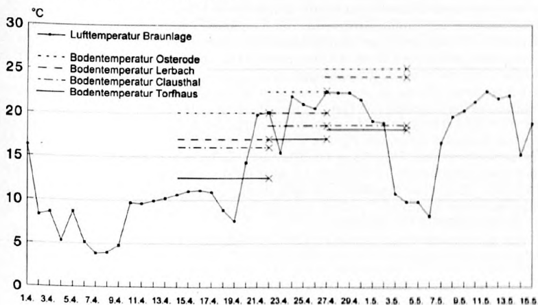
Abb. 2: Verlauf der Maximum-Temperaturen während des Kartierungszeitraumes. Darstellung wie in Abb. 1.
