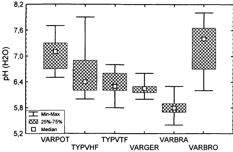
Abb. 3: Vergleich der Oberboden-pH-Werte (Untereinheiten des Arrhenatheretum elatioris im Aigoual-Massiv; s. Abb. 2).
