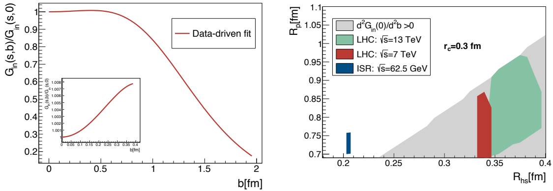
Abbildung 1: Links: Normalisierte Inelastizitätsdichte bei \sqrt{s} = 7 TeV wie aus den Daten extrahiert. Rechts: Hollowness Region (gefüllt-grau) und phänomenologisch kompatible Regionen mit ISR- und LHC-Daten in der (R_p, R_{hs}) -Ebene.
