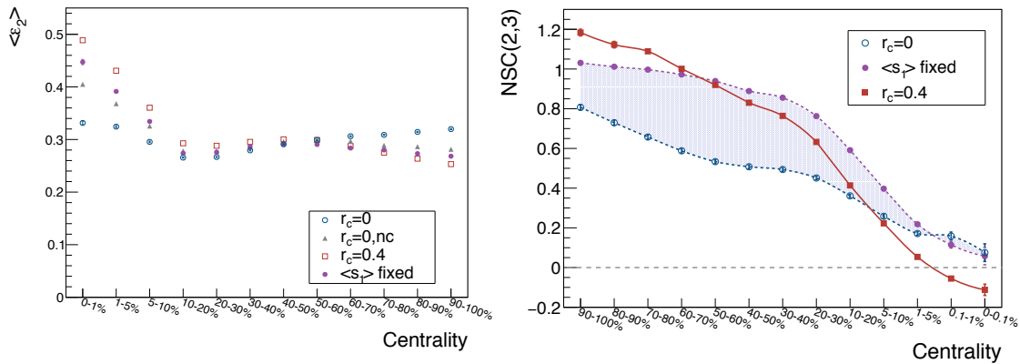
Abbildung 2: Links: Durchschnittswert der Exzentrizität in den korrelierten (rot leere Quadrate) und unkorrelierten Szenarien. Die verschiedenen Fälle von unkorreliert werden im Text erklärt. Rechts: Normierte symmetrische Kumulation als Funktion der Zentralität. Die hellviolette Bande enthält die unkorrelierten Ergebnisse, während die rote Linie dem korrelierten Szenario entspricht.
