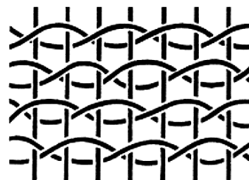
4 Gestaffeltes Zwirrbinden über ein passives System
