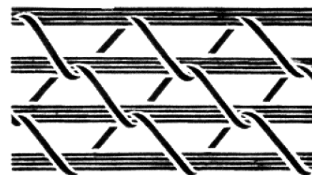
Durchstechend einhängendes Wulsthalbflechten
