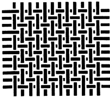
3 Dreibindiger, einseitiger Körper 1/2 bzw. 2/1
