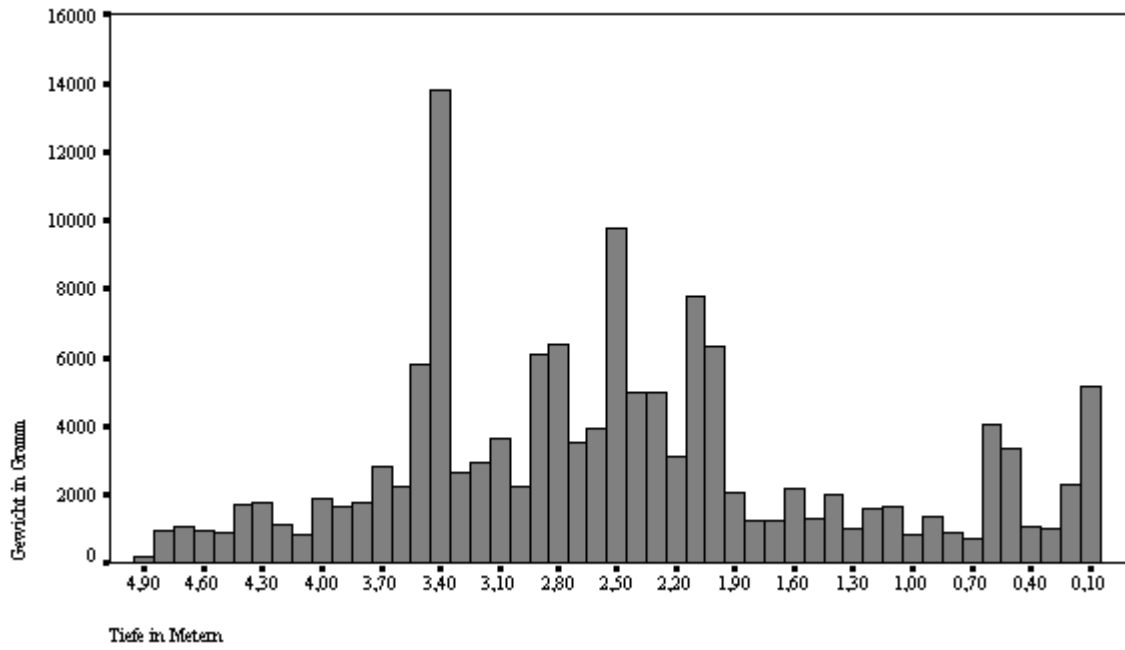
Abb. 8a Kursakata: Verteilung des Keramikgewichts
