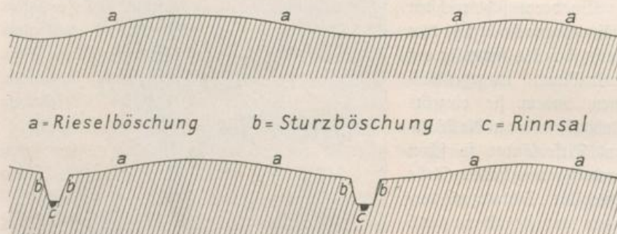
Die üblichen Böschungsformen der westafrikanischen Lateritlandschaft, schematische Darstellung. (Die Kanten bei b sind natürlich im allgemeinen durch Abwaschung abgerundet.)
