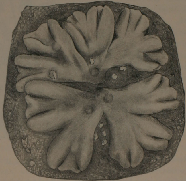
Abb. 1. Riccia glauca . Vergr. \frac{7}{1}
