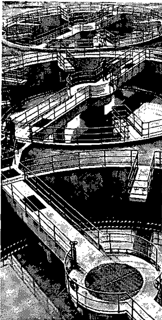
KW 1413 b
