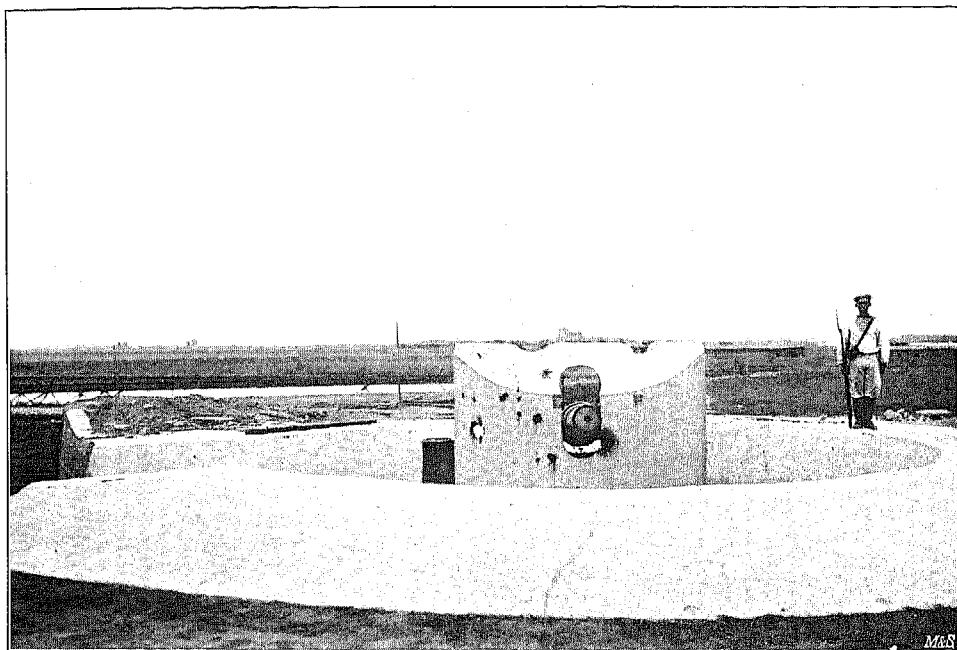
Kruppsches 12 cm Schnellladegeschütz auf dem nördlichen Flügel des Südforts mit 4 Vollkesseln und vielen Sprengkuchen.
