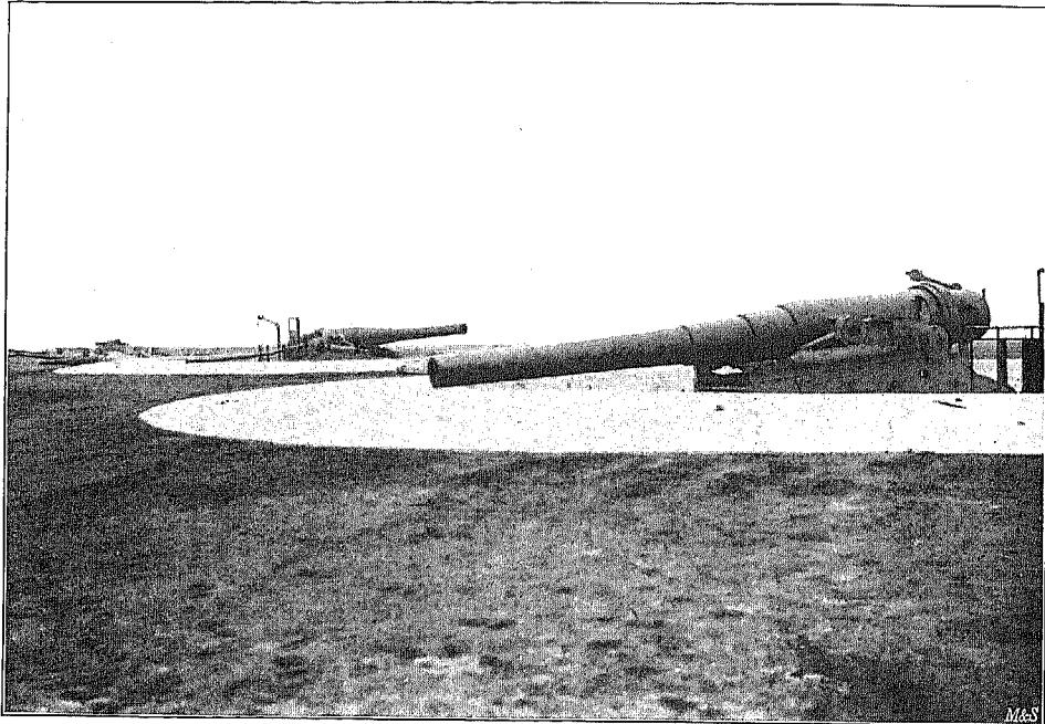
Strandbatterie. 2 Kruppsche 24 cm Geschütze, das erste nach See, das zweite landeinwärts auf den Peiljo gerichtet.
