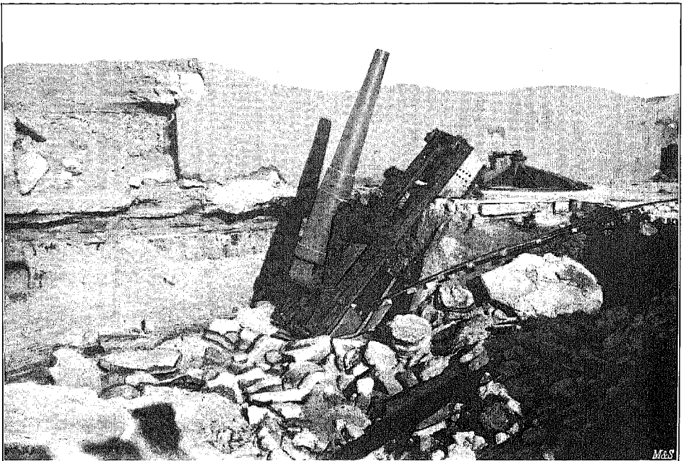
Ein Kruppsches 15 cm Geschütz L/22 neben dem südlichen Kavallerie des Südforts.
