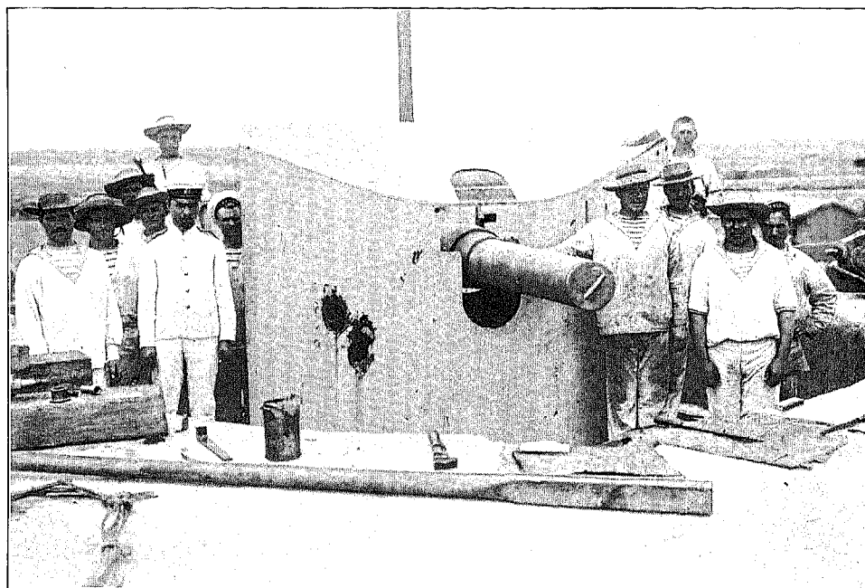
Kruppsches 12 cm Schnellladegeschütz auf dem nördlichen Kavallerie des Südforts mit 2 Vollkesseln und 1 Preller oben rechts am Schuttschild.
