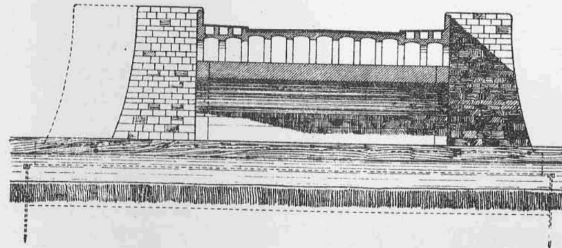
Schnitt C.
