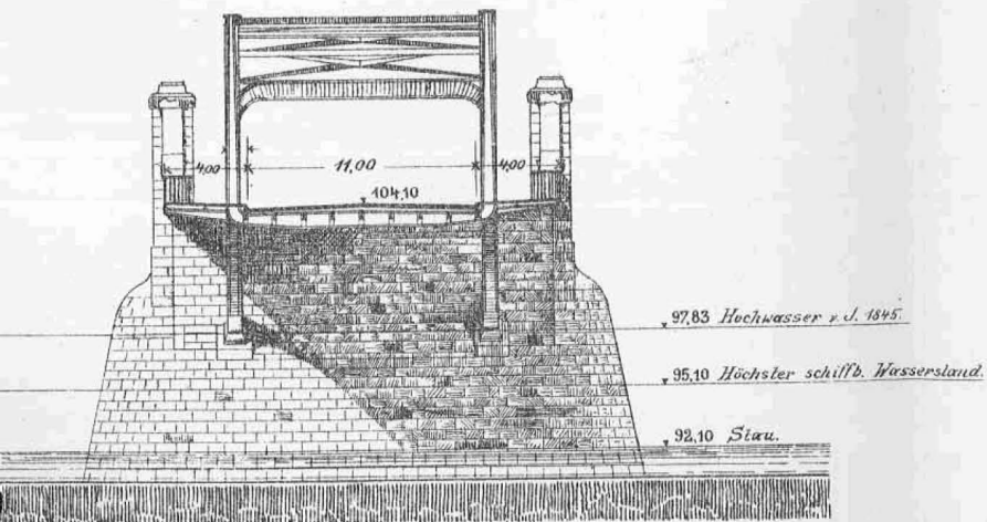
Schnitt E.
