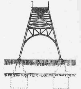
SEHNITT E.
