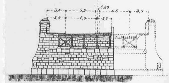
Schnitt durch die Mittelöffnung.
