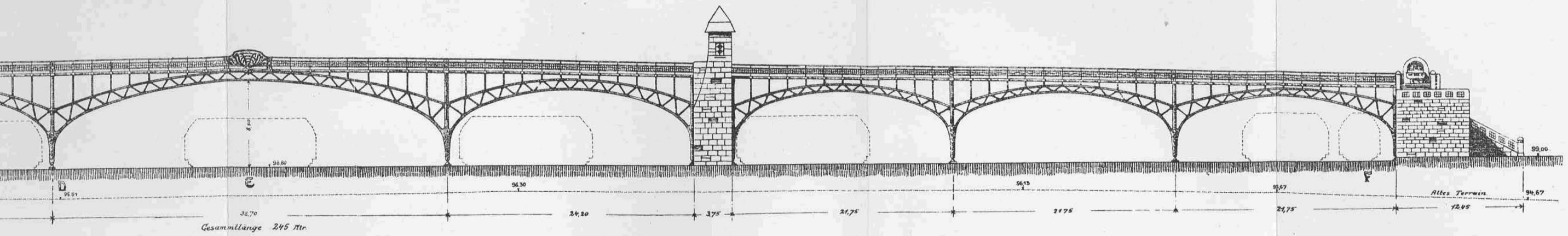
Schnitt C.
