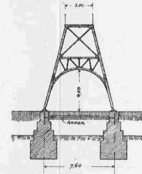
SEHNITT D.
