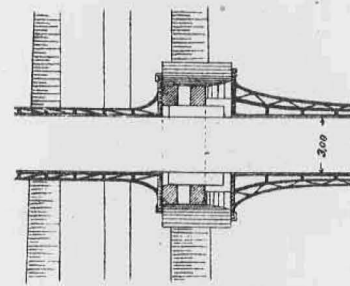
GRUNDRISS.
