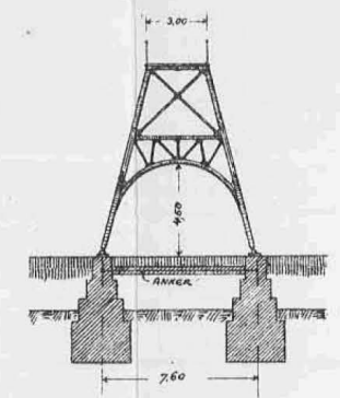
Schnitt D.
