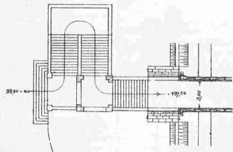
GRUNDRISS.
