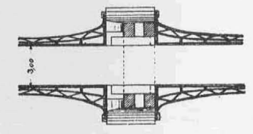
Grundriss.
