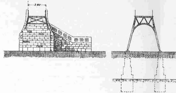
SEHNITT A.
