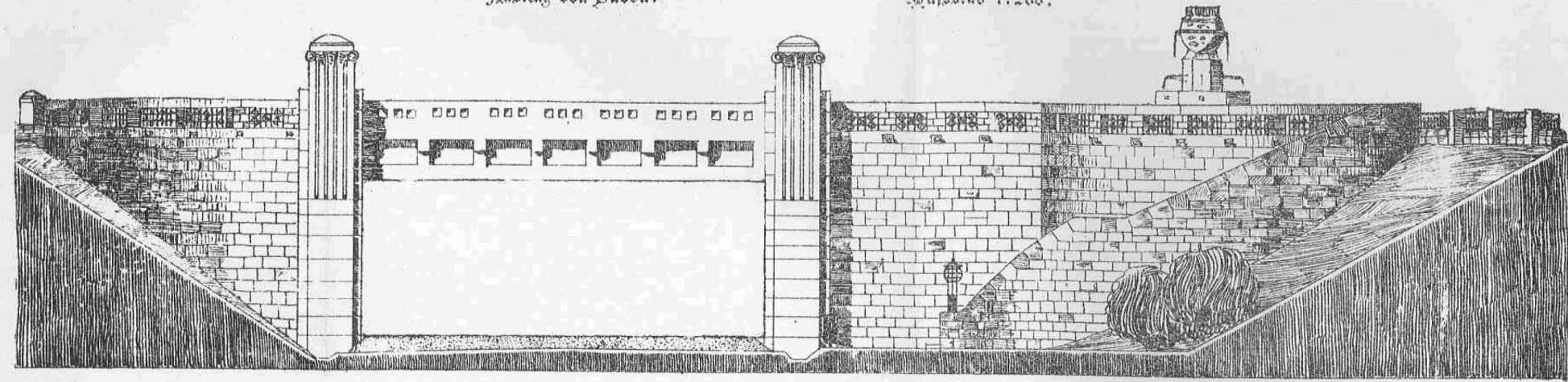
Ansicht von Süden.
