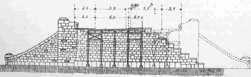
Schnitt durch die Seitenöffnung.
