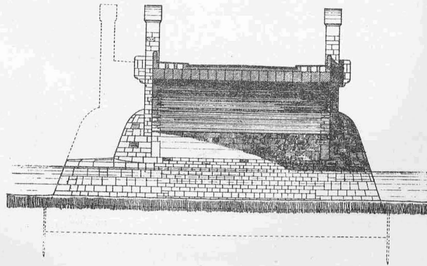
Schnitt A.
