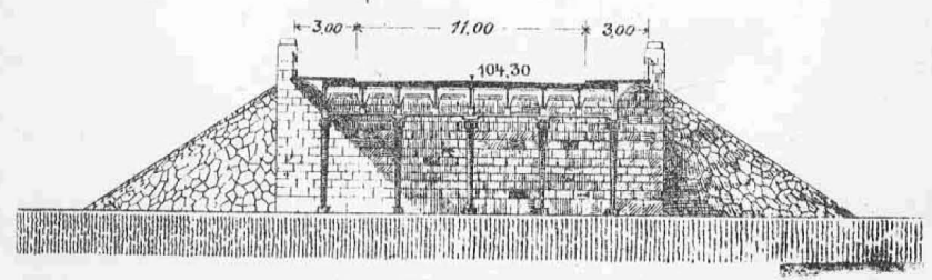
Schnitt A
