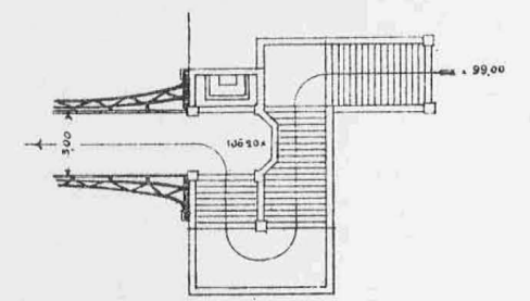
Grundriss.
