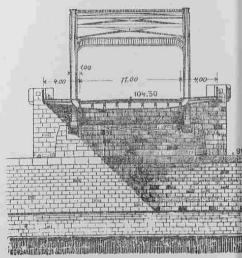
Schnitt C
