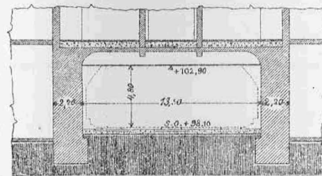
Schnitt e - f.
