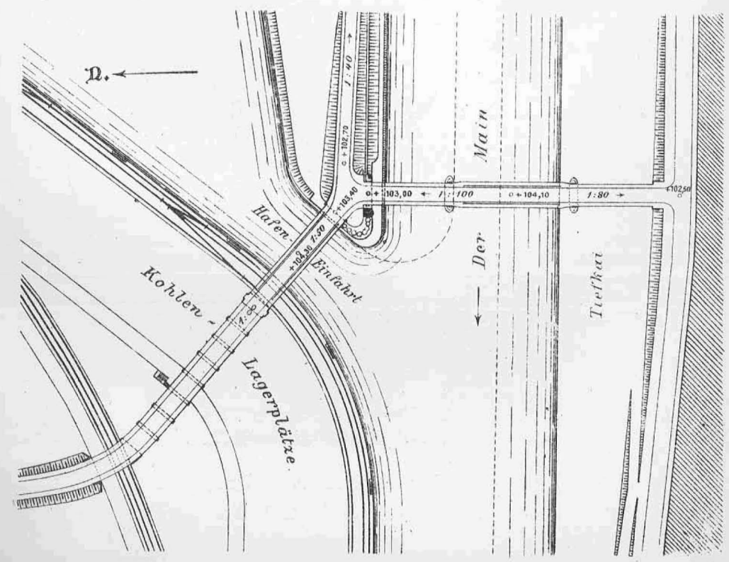
Maßstab = 1:4000.
