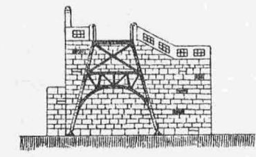
Schnitt F.
