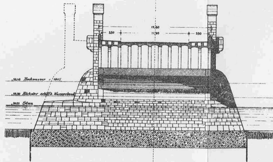
Schnitt B.
