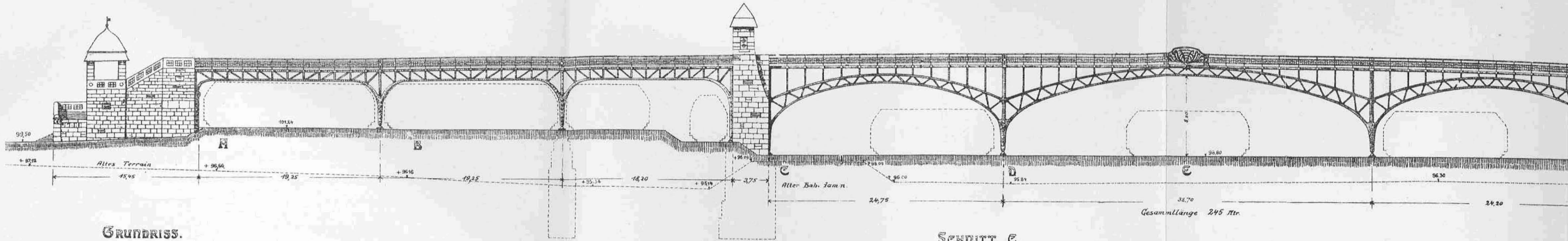
SEHNITT C.
