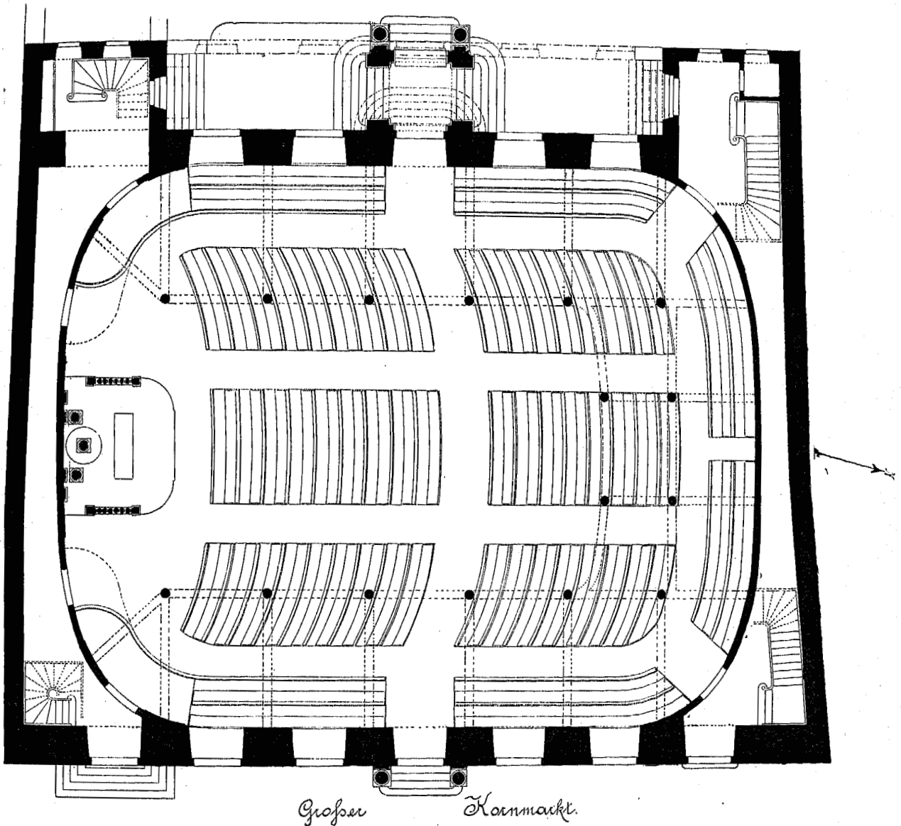
Fig. 290. Grundriss.
