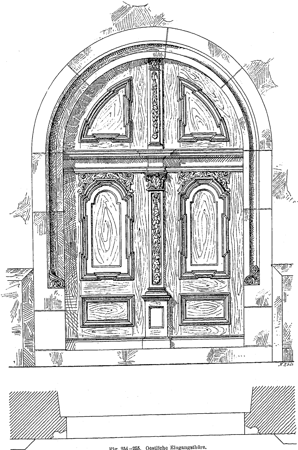
Fig. 254-255. Oestliche Eingangsthere.
