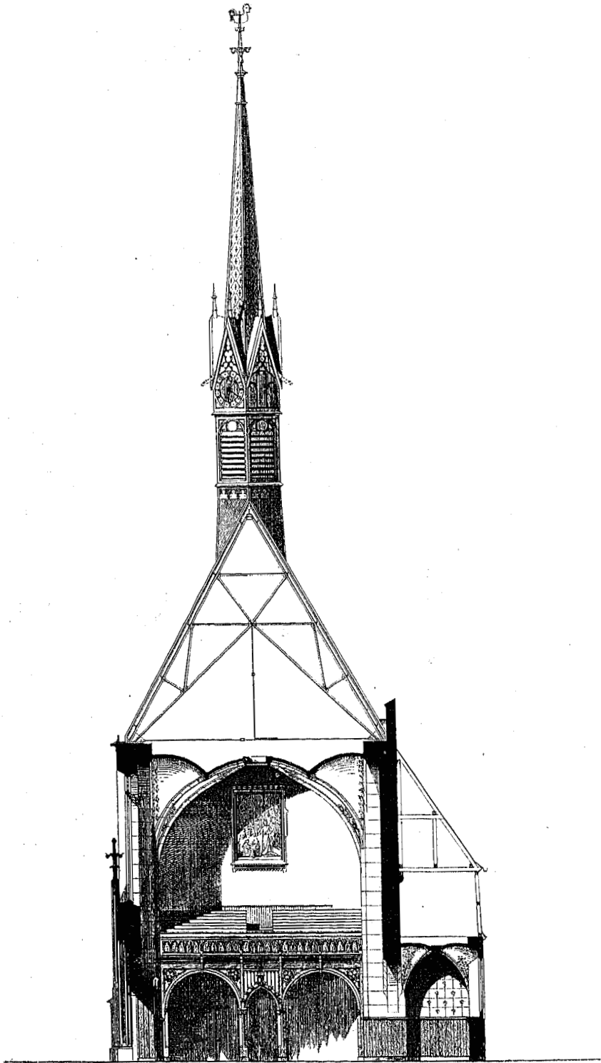
Fig. 139. Querschnitt.
