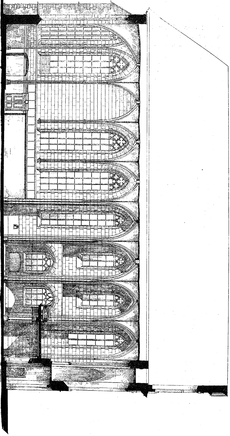
Fig. 214. Längenschnitt.
