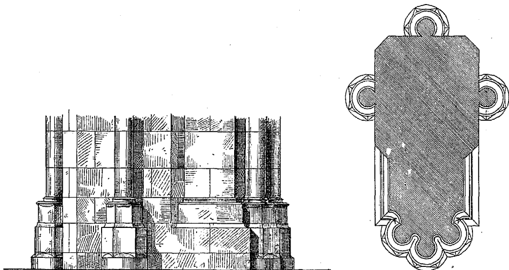
Fig. 72—73. Pfeiler zwischen Querschiff und Langhaus.
