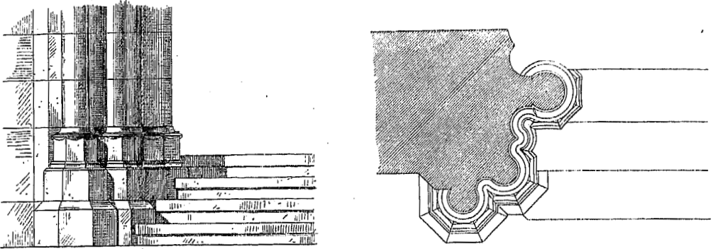
Fig. 68—69. Pfeiler an Triumphbogen.
