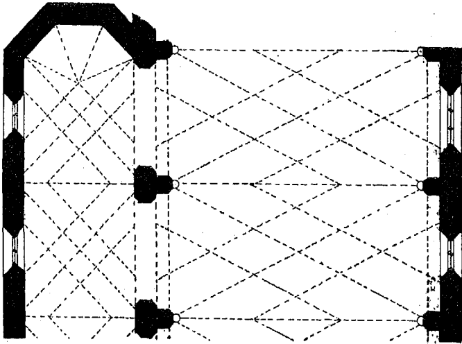
Fig. 329. Dreikönigs-Kirche; Gewölbesystem.
