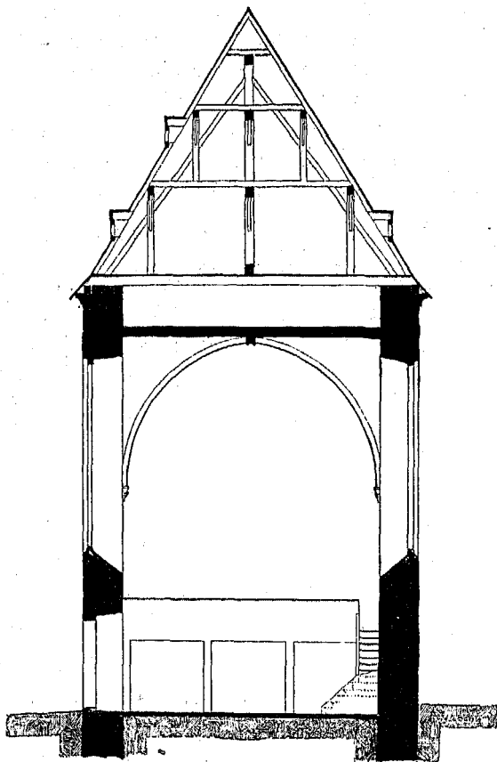
Fig. 307. Johanniter-Kirche; Querschnitt.
