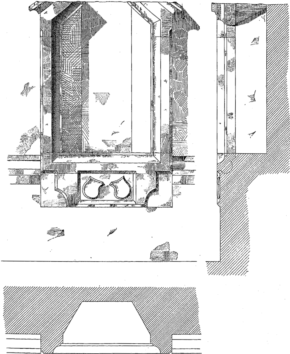
Fig. 192—194. Chornische.
