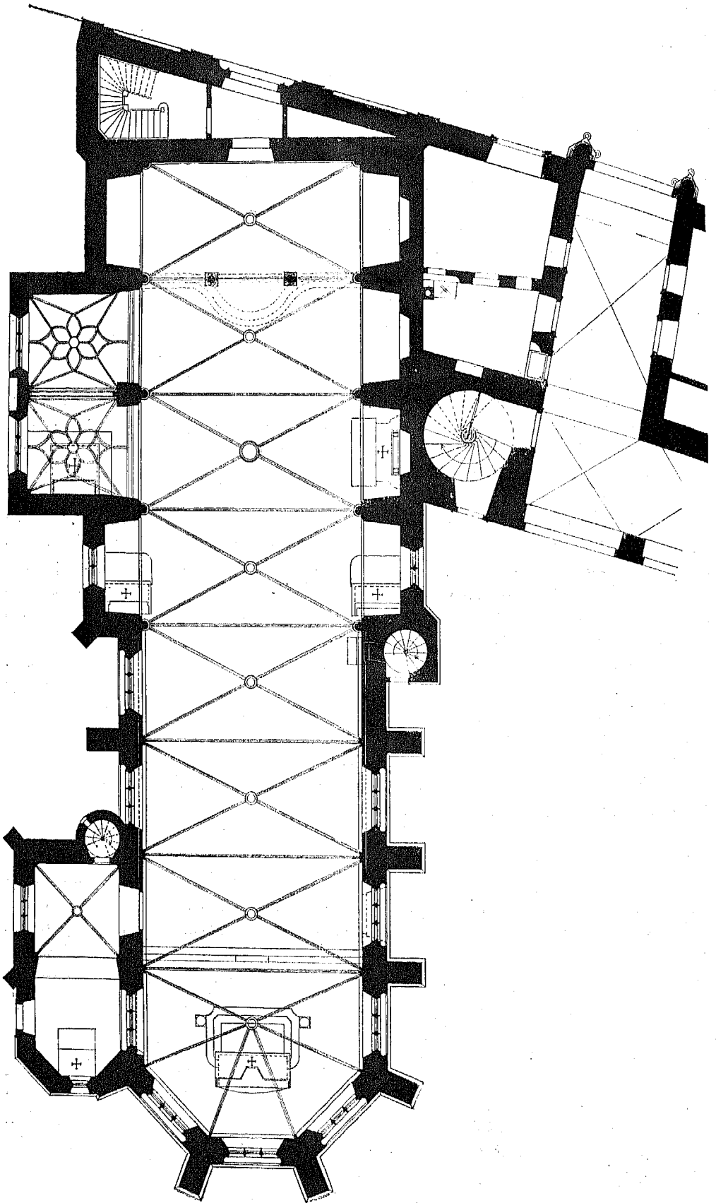
Fig. 211. Grundriss.
