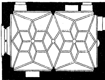
Fig. 234. Grundriss.
