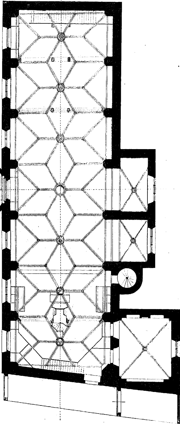
Fig. 135. Grundriss.
