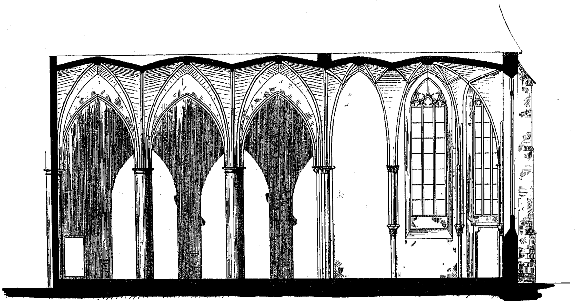
Fig. 88. Längenschnitt des östlichen Theils.
