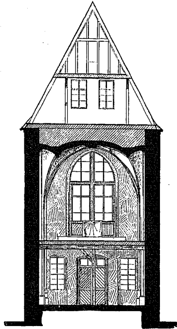
Fig. 236. Querschnitt.
