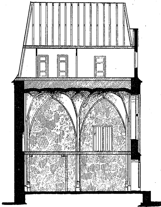
Fig. 237. Längenschnitt.
