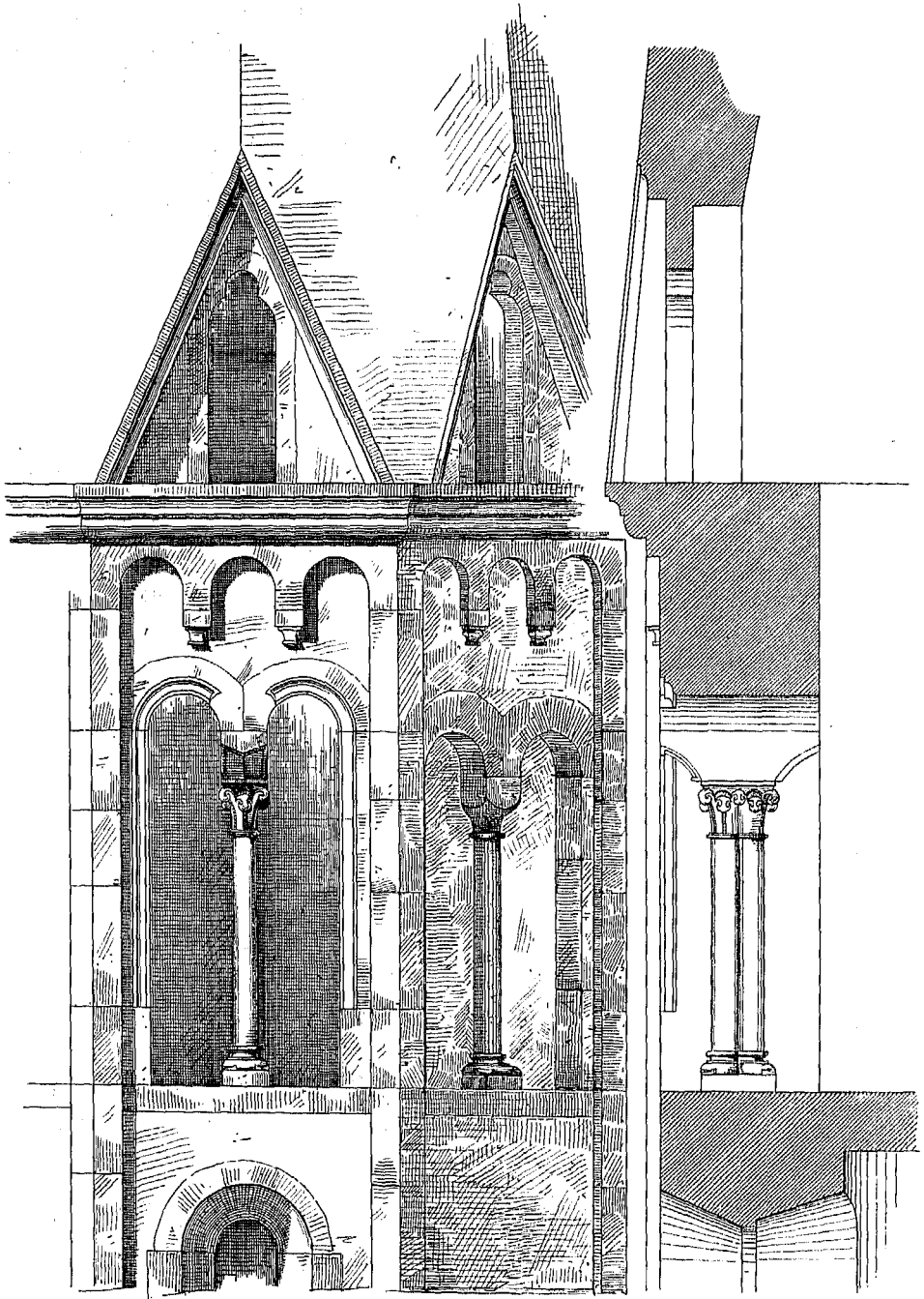
Fig. 7-8. Theile des Südthurms.
