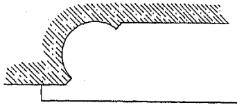
Fig. 243. Schlussstein.
