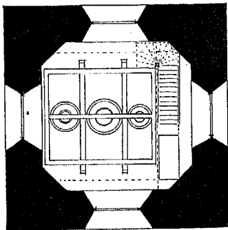
Fig. 258–259. Grundrisse des Thurmes.
