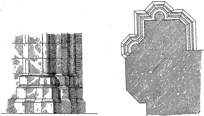
Fig. 70—71. Nordwestlicher Eckpfeiler an der Kapelle der heiligen Marla.
