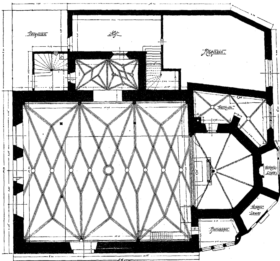
Fig. 171. Grundriss.
