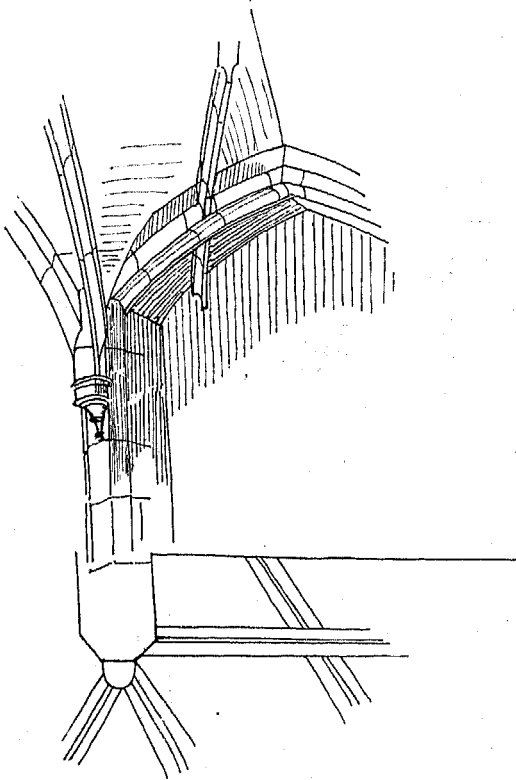
Fig. 331. Dreikönigs-Kirche; Gewölbeanfänger.
