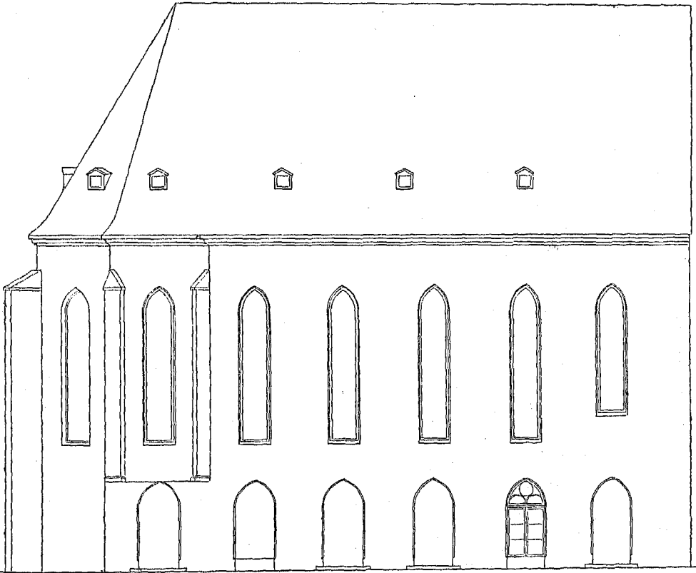
Fig. 310. Johanniter-Kirche; Nordseite.
