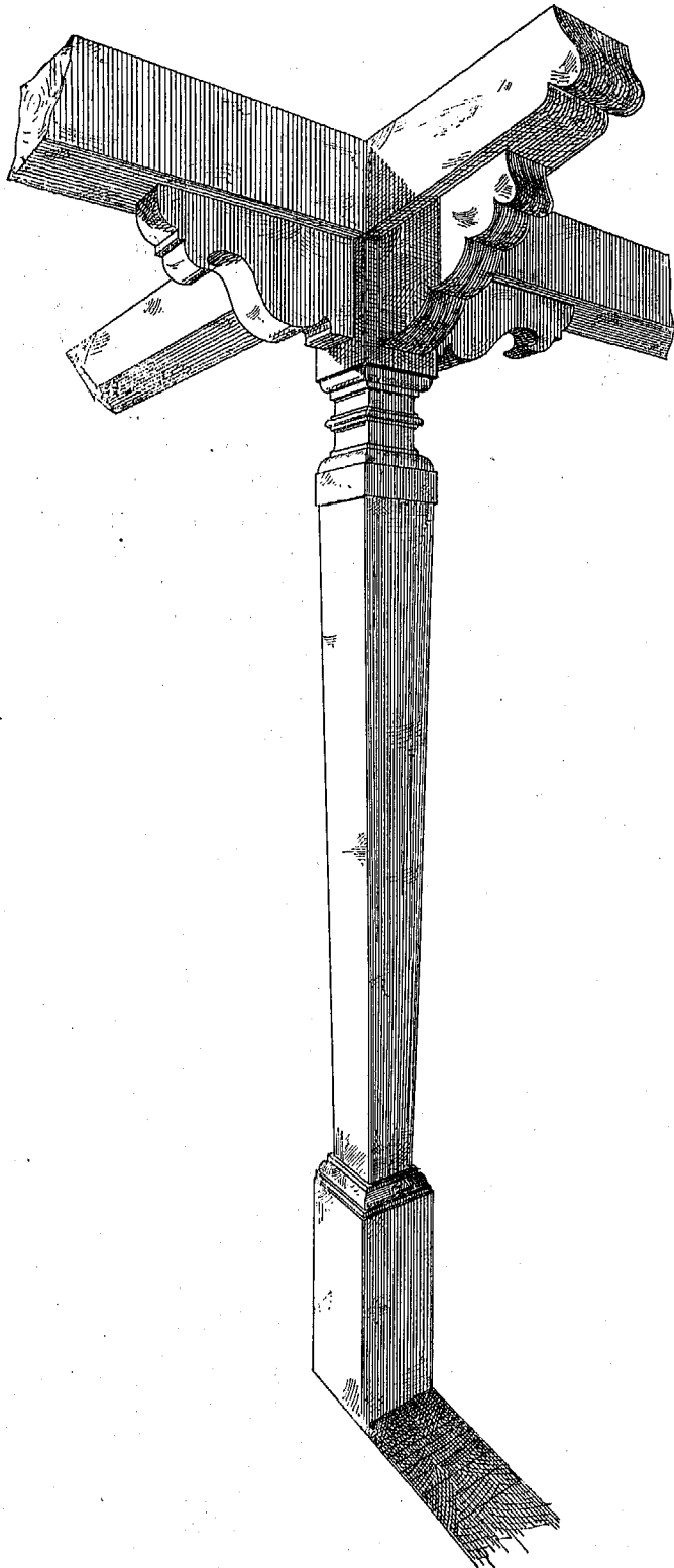
Fig. 185. Emporenstütze.
