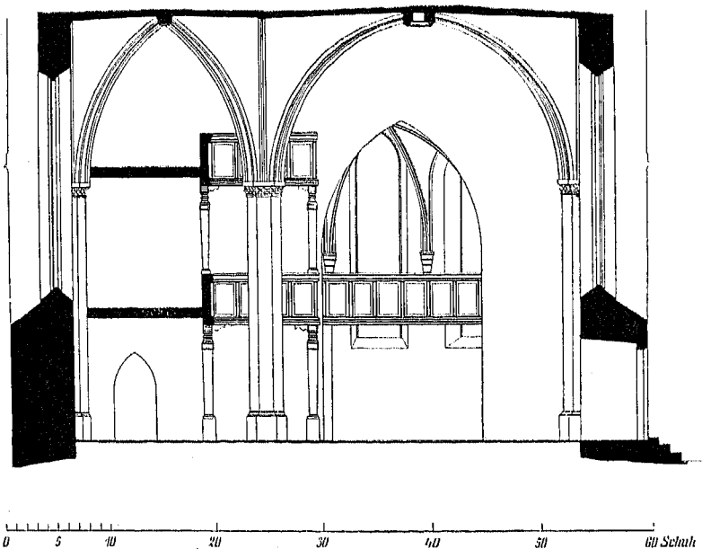
Fig. 48. Querschnitt.
