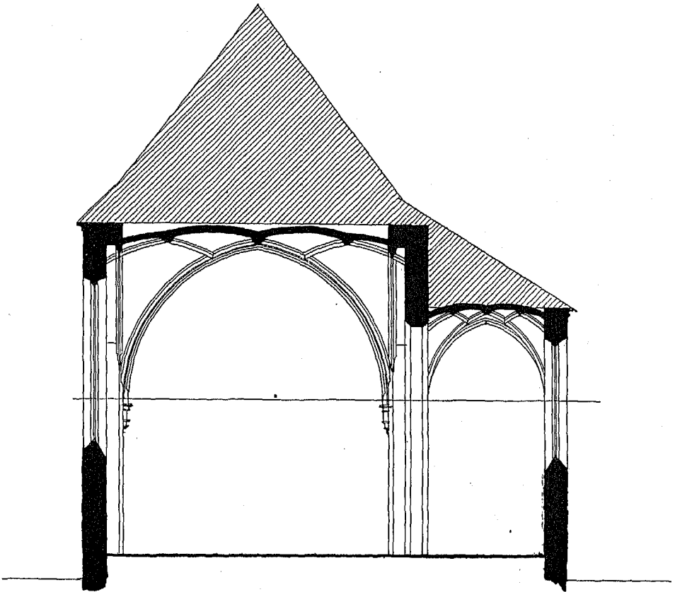
Fig. 330. Dreikönigs-Kirche; Querschnitt.
