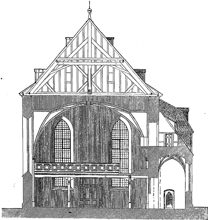
Fig. 174. Querschnitt.
