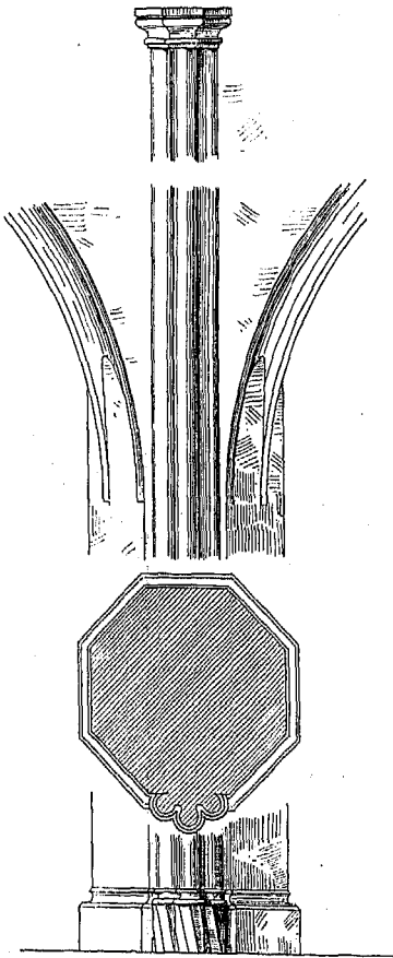
Fig. 18—21. Pfeiler im Langhaus.
