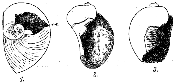
Naticopsis ampliata Phöll. Kohlenkalk von Visé. Etwas vergrössert.
