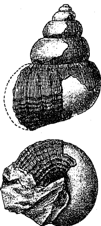
Flacilla sulcifera Hörnes sp. Subbullatusschicht, Sandling.
