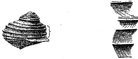
Sisenna turbinata Hörnes mut. Studeri Koken.
