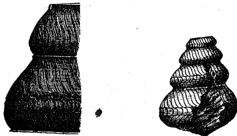
Pseudomurchisonia insueta Koken. (7:1 und 3:1.) Feuerkogel.
