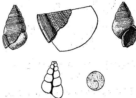
Ventricaria tumida Hörnes sp. Natürliche Grösse. Sandling.
