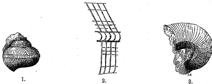
Euzone alauna Koken.
