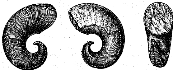
Pseudotubina biserialis Koken. (2:1.) Feuerkogel (?).
