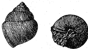
Bathycles acuminatus Koken. (4:1.) Feuerkogel.
