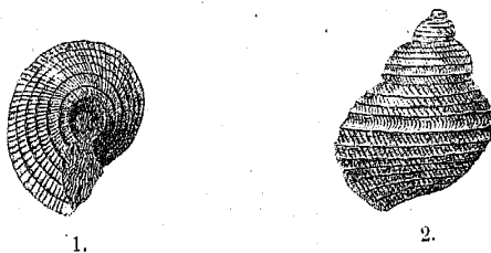
1. Sagana geometrica Koken. -- 2. Mittelform zwischen S. Hörnesi und S. geometrica .
