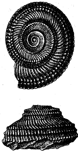
Solarium gradatum Koken. (4:1.) Feuerkogel.
