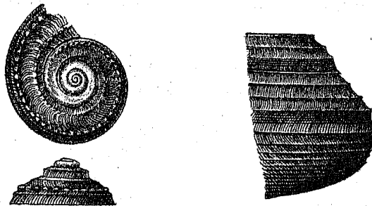
Sisenna turbinata Hörnes sp. Feuerkogel.
