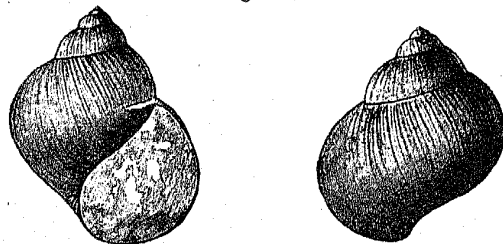
Neritaria (?) turbiniformis Koken. Etwa 3:1.
