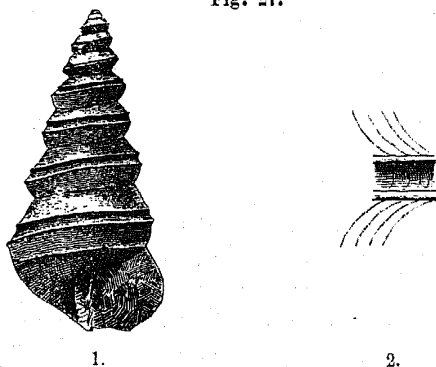
Murchisonia euglypha Koken. Vergrössert (6:1).
