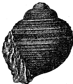
Ruffila denseincta Koken. Feuerkogel. In fünffacher Grösse.
