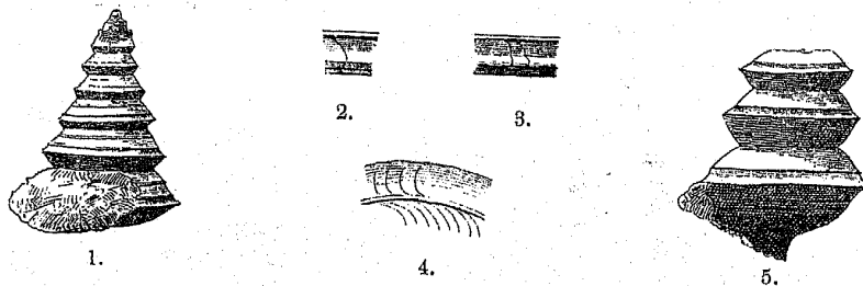
1., 2., 3. Vistilia Dittmari Koken.
