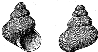
Acilia aequalis Koken. (2:1.) Röthelstein, ob. Schichten.
