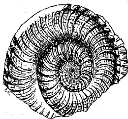
Anisostoma falcifer Koken. 5:1.
