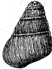
Rissoa torosa Koken. (3:1.) Feuerkogel.
