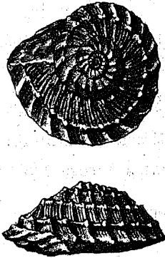
Visciana ornata Koken. (7:1.) Sommeraukogel.
