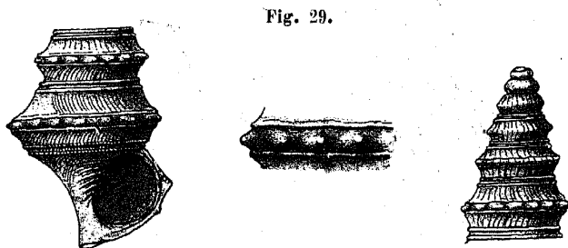
Verania cerithioides Koken. (7:1, das Schlitzband noch stärker vergrössert.) Feuerkogel.
