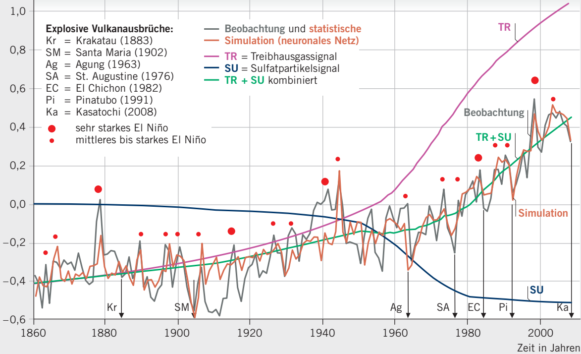
Die schwarze Kurve zeigt die aus Beobachtungsdaten abgeleiteten Anomalien (das heißt die Abweichungen vom Referenzmittelwert zwischen 1961 und 1990, der circa 15 °C beträgt) der global gemittelten bodennahen Lufttemperatur in den Jahren von 1860 bis 2008. Die rote Kurve zeigt die Reproduktion durch ein neuronales Netz, das 88 Prozent der beobachteten Varianz erklärt. Einige durch Vulkanausbrüche verursachte Abkühlungs- und durch El-Niño-Ereignisse verursachte Erwärmungsperioden sind markiert. Die violette Kurve (TR) zeigt die Erwärmung durch die anthropogen angestiegenen Treibhausgaskonzentrationen, die blaue (SU) die Abkühlung durch die ebenfalls anthropogenen erhöhten Sulfatpartikelkonzentrationen. Die grüne Kurve ist der kombinierte anthropogene Effekt, der offenbar eine Erwärmung um rund 0,8 °C anzeigt.
