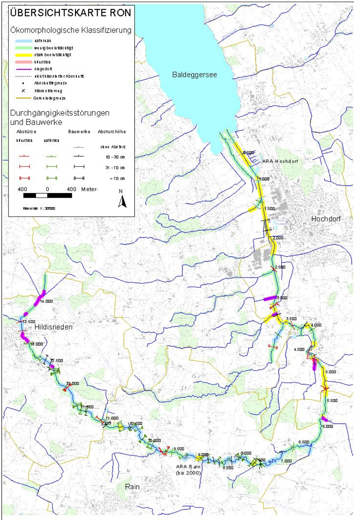
Abbildung 15: Ökomorphologischer Zustand der Ron (Rappo, 2001). Die Lage und Absturzhöhe von natürlichen und künstlichen Abstürzen ist angegeben.
