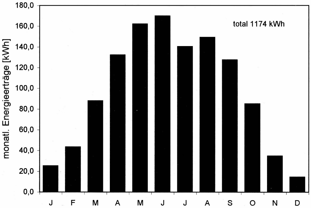
Abb. 4: Monatliche Erträge der Photovoltaikanlage (kWh).
