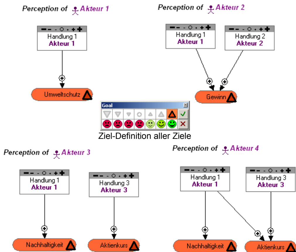
Abbildung A.28: Beispiel-case „Nachhaltigkeit“ zur Erläuterung des Fehlers im Analysetool Rating of Tactics mit den Wahrnehmungsgraphen der Akteure 1, 2, 3 und 4 in einer arena
