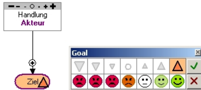
Abbildung A.15: Wahrnehmungsgraph für die Erläuterung des Zufriedenheits- und Frustrationswertes in DANA
