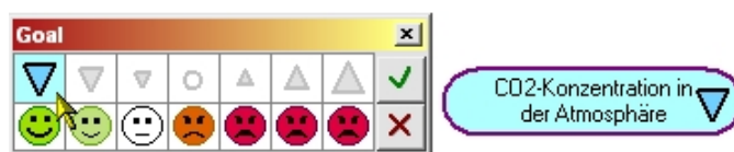
Abbildung A.5: Beispiel für die Zieldefinition „Rückgang der CO 2 -Konzentration in der Atmosphäre“ in DANA
