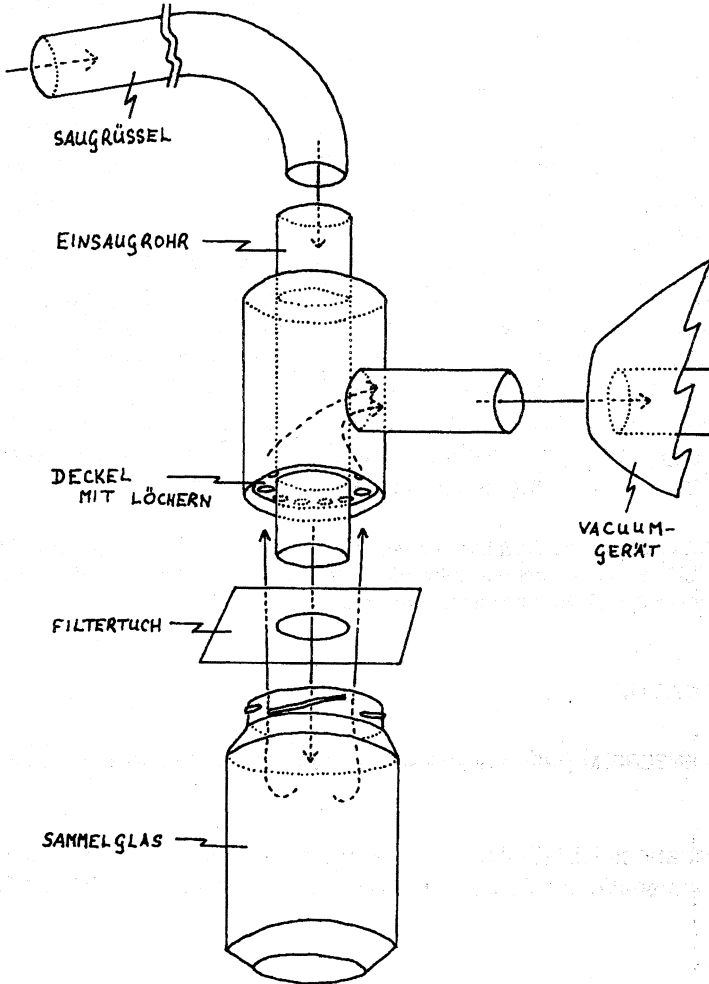
Abb. 2 Auseinandergezogene Darstellung des Exhaustors. Die Pfeile geben die Richtung der Luftbewegung an.
