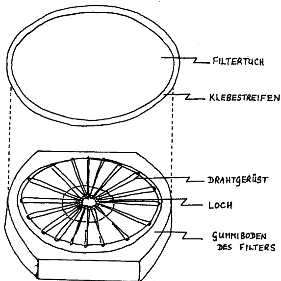
Abb. 1 Filtergerüstkonstruktion des Vakuumerätes
