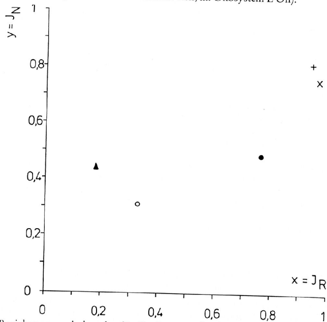
Abb. 2: Beziehungen zwischen den für die einzelnen Ökosysteme bestimmten Reaktionszahlen-Indices ( I_R ) und den Stickstoffzahlen-Indices ( I_N ).
