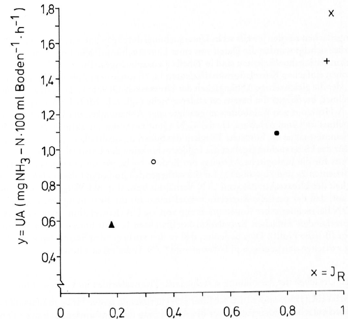
Abb. 4: Beziehungen zwischen den für die einzelnen Ökosysteme bestimmten Reaktionszahlen-Indices ( I_R ) und den mittleren Ureaseaktivitäten im humosen A-Horizont.
