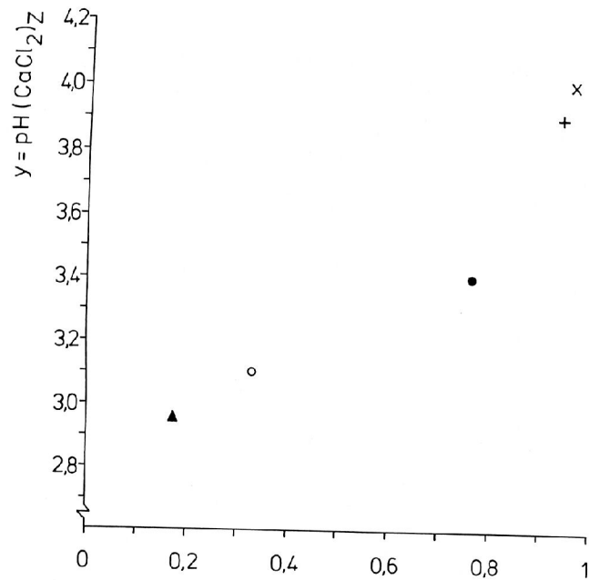
Abb. 1: Beziehungen zwischen den für die einzelnen Ökosysteme bestimmten Reaktionszahlen-Indices ( I_R ) und den zentralen \text{pH}(\text{CaCl}_2) -Werten des Bodens im Hauptwurzelbereich der Kräuter (in den Ökosystemen A bis D Ah bzw. Aeh, im Ökosystem E Oh).
