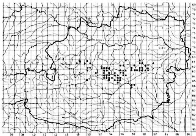
Abb. 1: Das Areal von Festuca versicolor .
