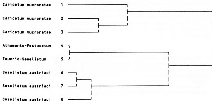
Abb. 5: Clusteranalyse (CLC mit similarity ratio SR) von 9 Lokal-Tabellen des Caricetum mucronatae (1–3), Athamanto-Festucetum (4), Teucrio-Seselietum (5) und Seselietum austriaci (6–9). Die Fusionskala ist in diesem Diagramm als Unähnlichkeit (1-SR) angegeben. Für die nähere Identifikation der Lokal-Tabellen siehe Tab. 3.
