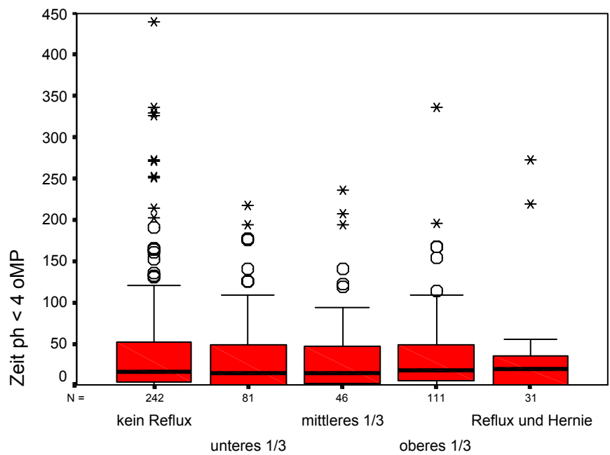
Abbildung 10: Zeit in der pH<4 am oMP bei zunehmender Höhe des Reflexes in der oMDP
