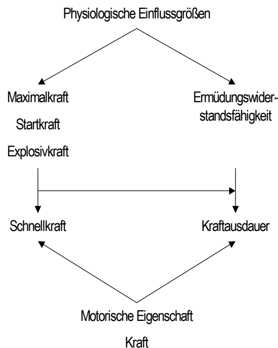
Abb. 1: Einflussgrößen des Kraftverhaltens (modif. n. GÜLLICH/SCHMIDTBLEICHER 1999, 224)
