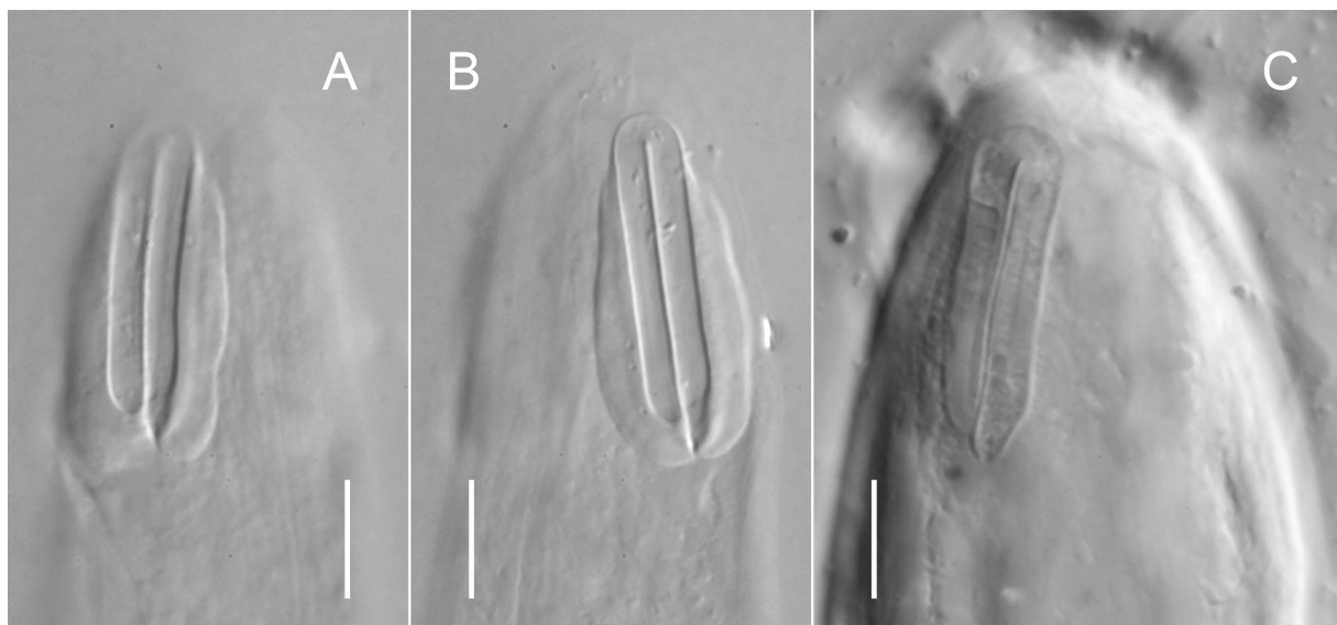
Fig. 15. A–B. Anterior end of the holotype of Diplopeltis ovalis Ditlevsen, 1928. C. Anterior end of the lectotype of Diplopeltis asymmetricus Allgén, 1935. Scale bar = 10 \mu\text{m} .
