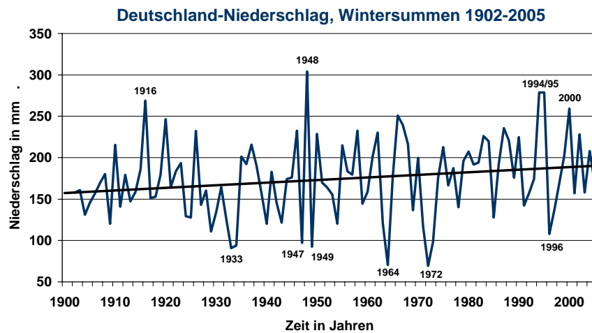
Abb. 15. Ähnlich Abb. 14, jedoch Winter.
