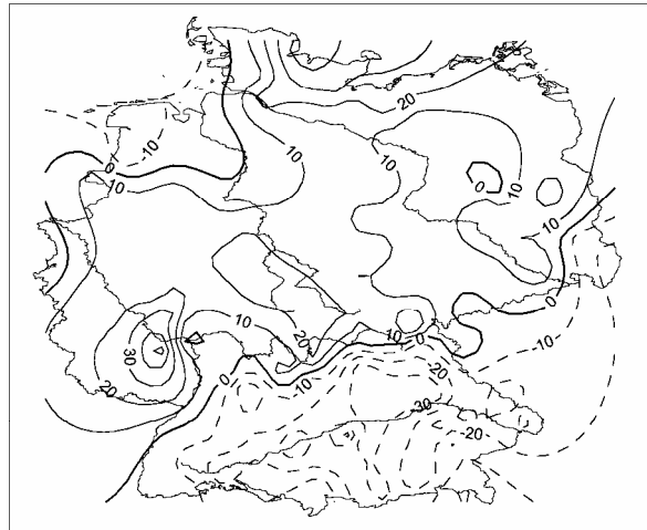
Niederschlag Relativer Trend [% des Mittelwertes] mit signifikanten Gebieten Januar 1961-1990
