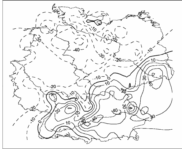
Niederschlag Relativer Trend [% des Mittelwertes] mit signifikanten Gebieten August 1971-2000
