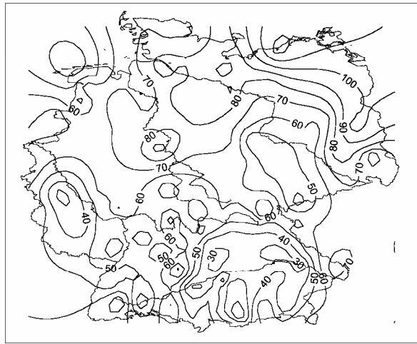
Niederschlag Relativer Trend [% des Mittelwertes] mit signifikanten Gebieten März 1971-2000
