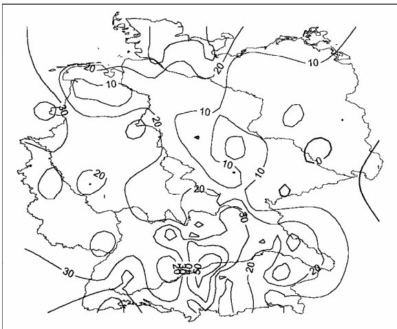
Niederschlag Relativer Trend [% des Mittelwertes] mit signifikanten Gebieten Winter 1901-2000
