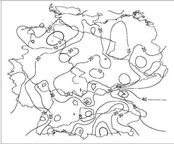
Niederschlag Relativer Trend [% des Mittelwertes] mit signifikanten Gebieten Januar 1901-2000
