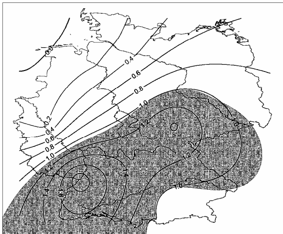
Lufttemperatur Linearer Trend [k] mit signifikanten Gebieten Sommer 1961-1990
