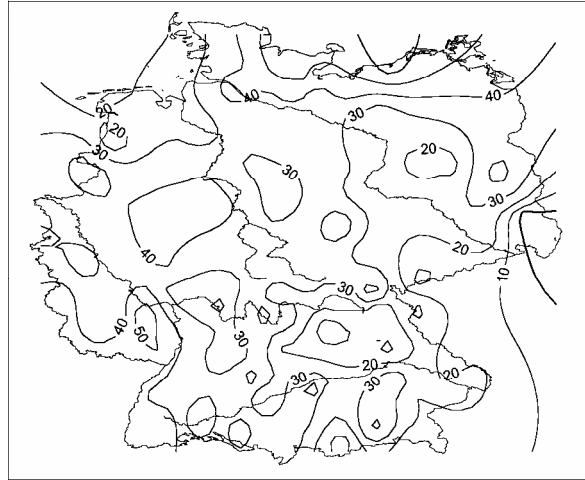
Niederschlag Relativer Trend [% des Mittelwertes] mit signifikanten Gebieten Januar 1971-2000
