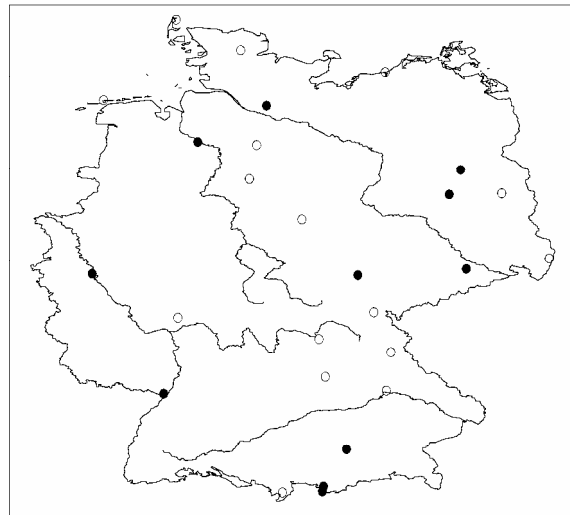
Abb. 3. Temperaturdaten-Stationsnetz, wie es der Trendanalyse zugrunde liegt. Mit leeren Kreisen sind die Stationen gekennzeichnet, von denen Daten nur für 1951-2000 vorliegen (vgl. Tab. 1).
