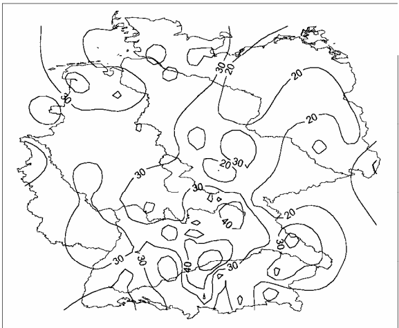
Niederschlag Relativer Trend [% des Mittelwertes] mit signifikanten Gebieten Dezember 1901-2000
