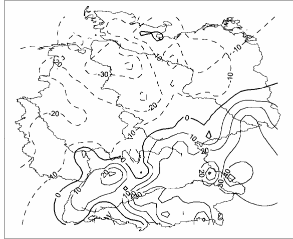
Niederschlag Linearer Trend [mm] mit signifikanten Gebieten August 1971-2000
