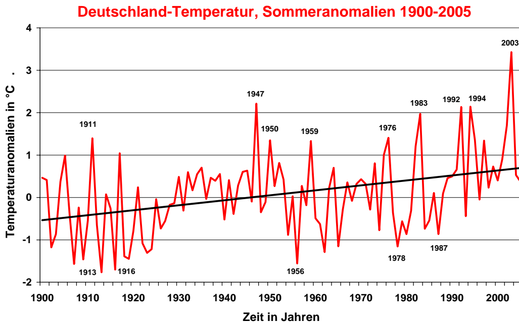
Abb. 11. Sommeranomalien (Juni, Juli, August) 1900-2005 (relativ zu 1961-1990) des Gebietsmittels der bodennahen Lufttemperatur in Deutschland mit linearem Trend (Datenquelle wie Abb. 9).
