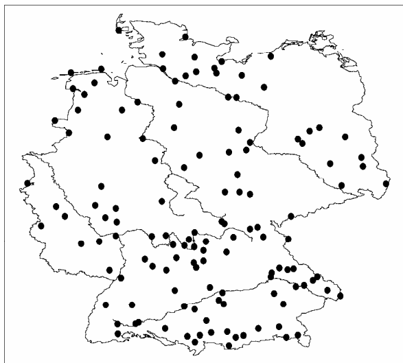
Abb. 4. Ähnlich Abb. 3, jedoch Niederschlag.
