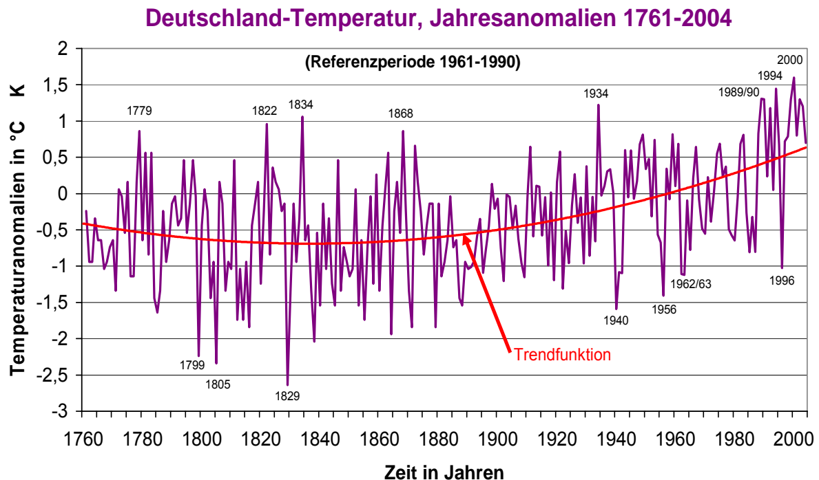
Abb. 10. Jahresanomalien 1761-2004 (relativ zu 1961-1990) des Gebietsmittels der bodennahen Lufttemperatur in Deutschland mit nicht-linearer Trendfunktion, die jedoch ab 1901 (vgl. Tab. 2) in guter Näherung linear ist und eine Erwärmung um rund 1\text{ °C} anzeigt (Datenquelle: Rapp, 2000, ergänzt nach DWD).
