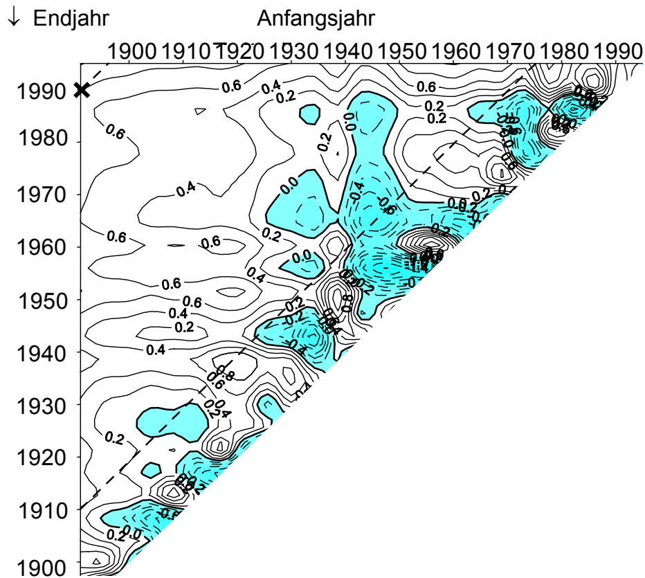
Abb. 9. Trendmatrix der bodennahen Lufttemperatur, Flächenmittel Deutschland; Erklärung siehe Text (nach Rapp, 2000).
