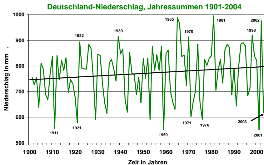
Abb. 13. Jahressummen 1901-2004 des Gebietsniederschlags Deutschland (Datenquelle: DWD) mit linearem Trend.
