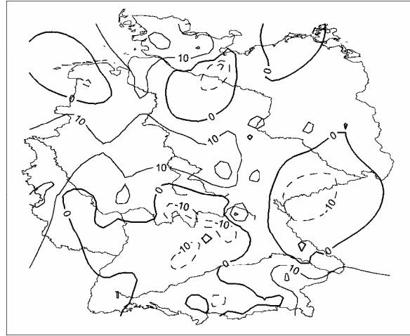
Niederschlag Relativer Trend [% des Mittelwertes] mit signifikanten Gebieten Jahr 1971-2000
