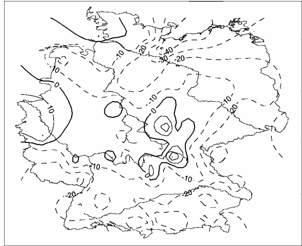
Niederschlag Relativer Trend [% des Mittelwertes] mit signifikanten Gebieten Herbst 1971-2000
