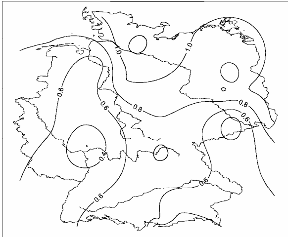
Lufttemperatur Linearer Trend [K] mit signifikanten Gebieten Sommer 1901-2000
