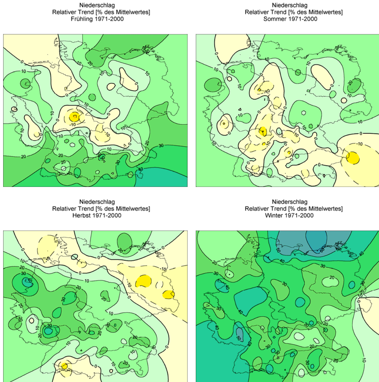
Abb. 19. Ähnlich Abb. 18, jedoch 1971-2000.
