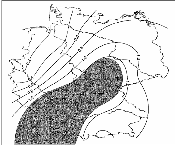
Lufttemperatur Linearer Trend [K] mit signifikanten Gebieten Herbst 1961-1990
