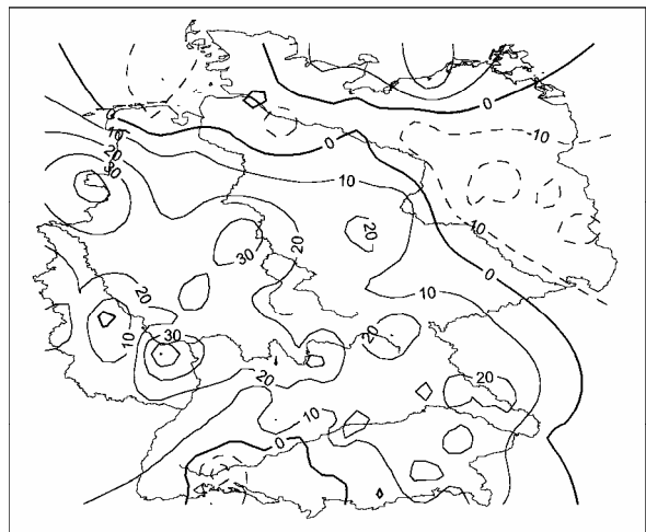
Niederschlag Relativer Trend [% des Mittelwertes] mit signifikanten Gebieten Winter 1931-1960
