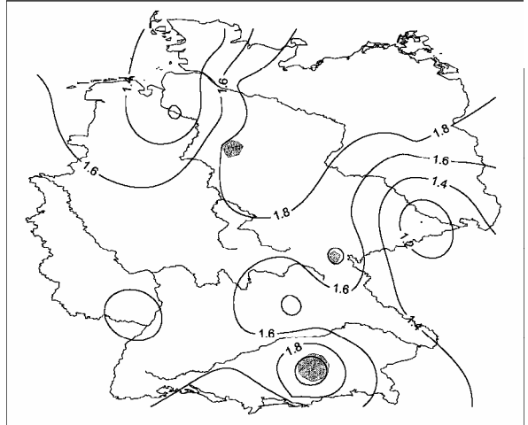
Lufttemperatur Linearer Trend [K] mit signifikanten Gebieten Sommer 1931-1960
