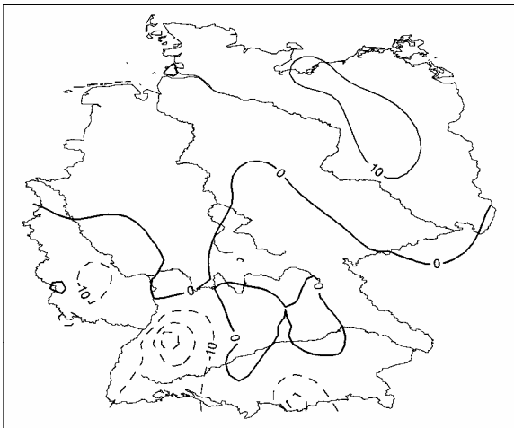
Sonnenscheindauer Linearer Trend [h] mit signifikanten Gebieten Dezember 1951-2000
