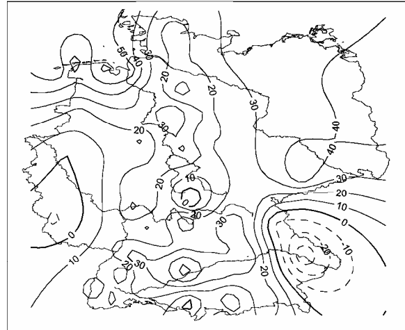
Sonnenscheindauer Linearer Trend [h] mit signifikanten Gebieten Januar 1971-2000
