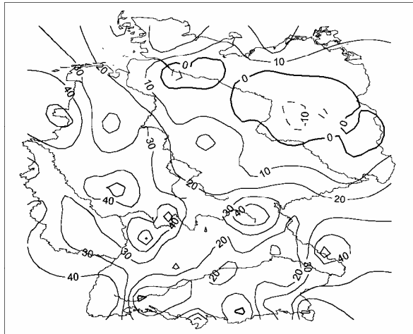
Niederschlag Linearer Trend [mm] mit signifikanten Gebieten September 1971-2000
