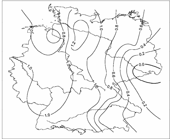
Lufttemperatur Linearer Trend [K] mit signifikanten Gebieten August 1971-2000
