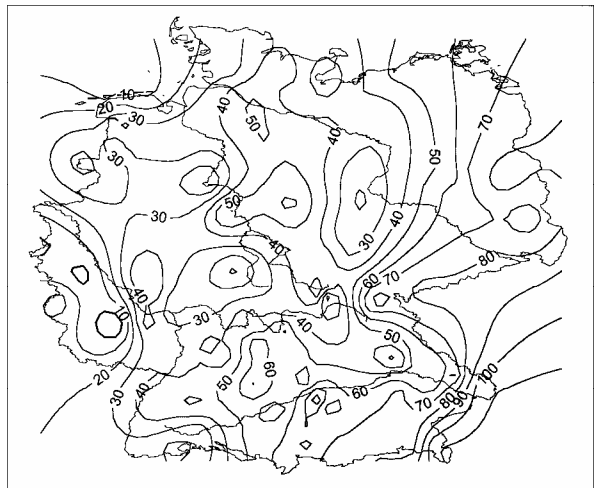
Niederschlag Relativer Trend [% des Mittelwertes] mit signifikanten Gebieten April 1971-2000
