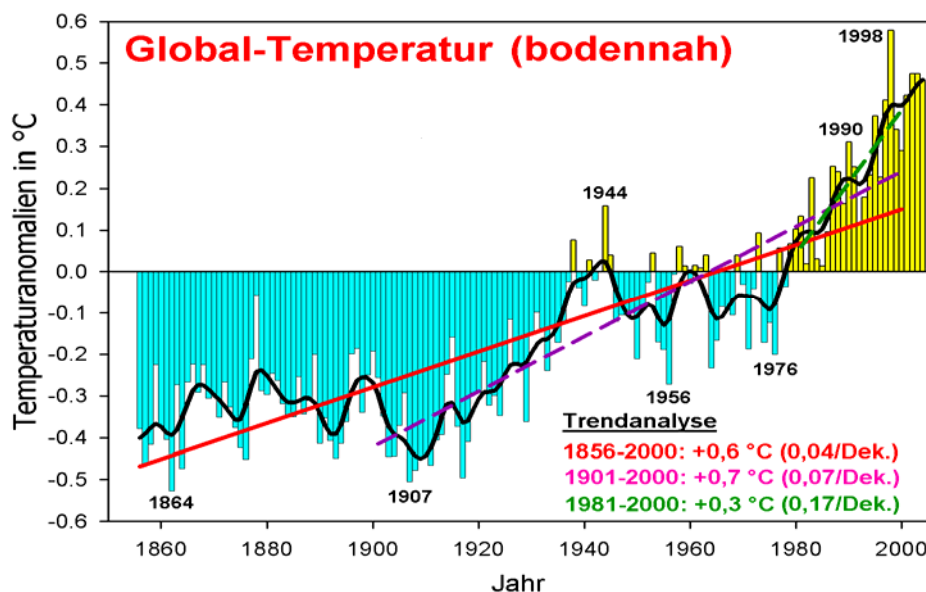
Abb. 1. Global gemittelte Jahresanomalien 1856-2004 (relativ zu 1961-1990) der bodennahen Lufttemperatur, Säulen, mit 10-jährig geglätteten Daten, schwarze Kurve, und Trendanalysen (Datenquelle: Jones et al., 1999; CRU, 2005, bearbeitet).
