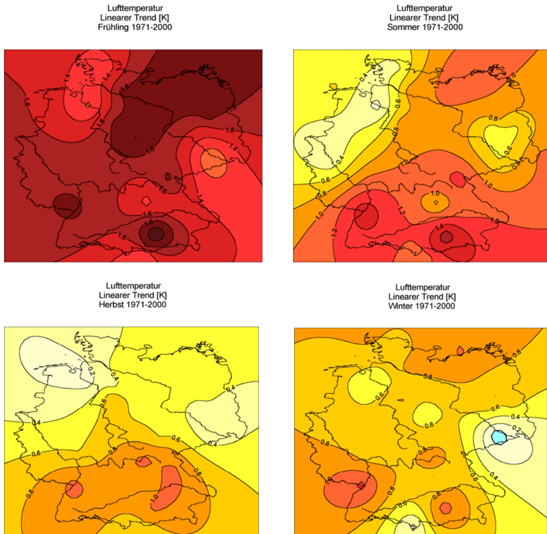
Abb. 17. Ähnlich Abb. 16, jedoch 1971-2000.
