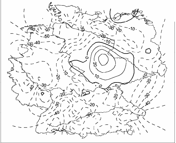
Niederschlag Relativer Trend [% des Mittelwertes] mit signifikanten Gebieten Dezember 1971-2000
