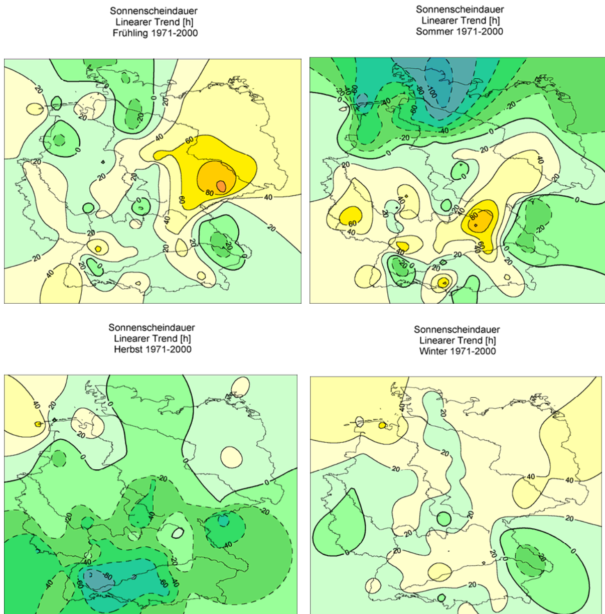
Abb. 20. Karten der linearen Sonnenscheindauer-Trends 1971-2000 in Stunden, alle Jahreszeiten (gelblich Zunahme, grünlich/Bläulich Abnahme).
