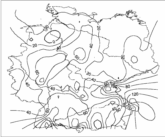
Niederschlag Linearer Trend [mm] mit signifikanten Gebieten Januar 1901-2000
