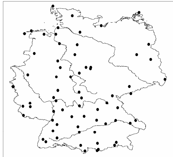
Abb. 5. Ähnlich Abb. 3, jedoch Sonnenscheindauer.
