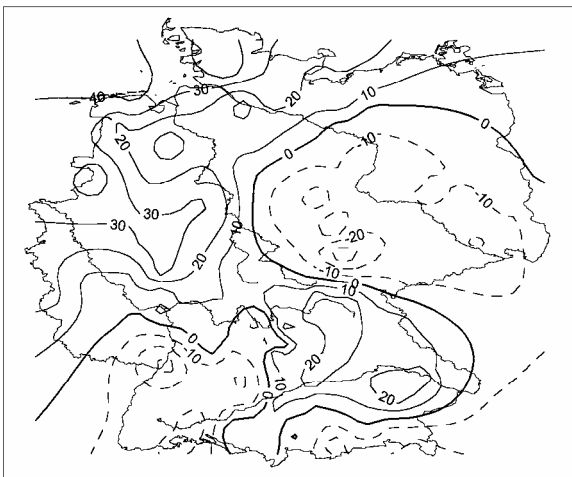
Niederschlag Relativer Trend [% des Mittelwertes] mit signifikanten Gebieten September 1901-2000
