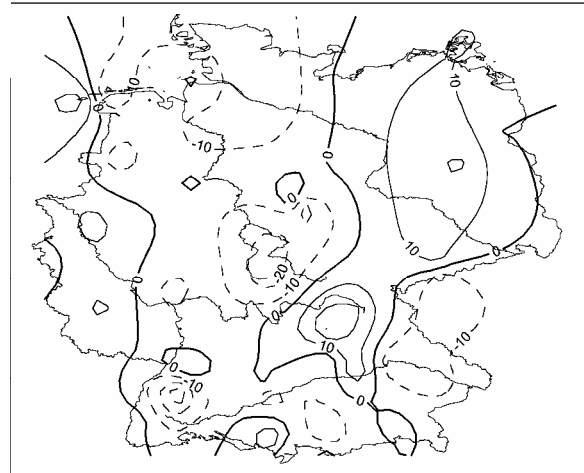
Sonnenscheindauer Linearer Trend [h] mit signifikanten Gebieten Juli 1971-2000
