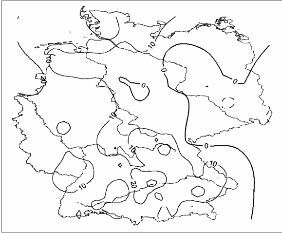
Niederschlag Relativer Trend [% des Mittelwertes] mit signifikanten Gebieten Jahr 1961-1990
