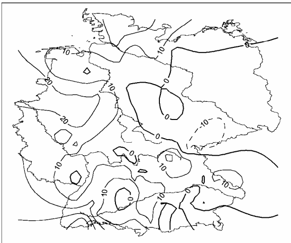
Niederschlag Linearer Trend [mm] mit signifikanten Gebieten Januar 1931-1960
