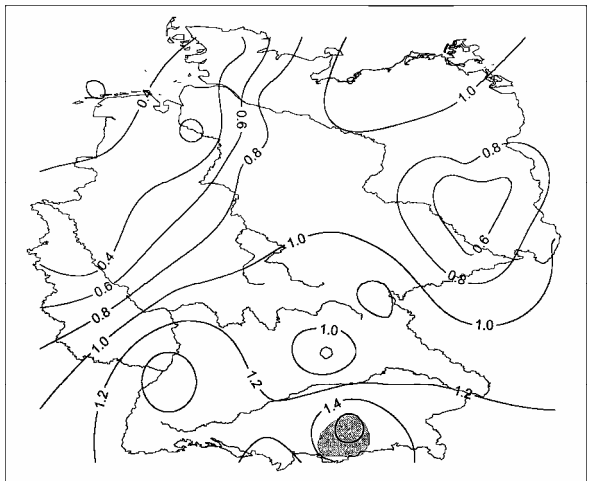
Lufttemperatur Linearer Trend [k] mit signifikanten Gebieten Sommer 1971-2000
