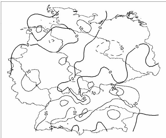
Niederschlag Relativer Trend [% des Mittelwertes] mit signifikanten Gebieten Frühling 1901-2000
