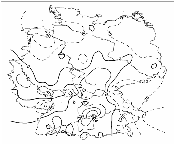
Niederschlag Relativer Trend [% des Mittelwertes] mit signifikanten Gebieten April 1901-2000
