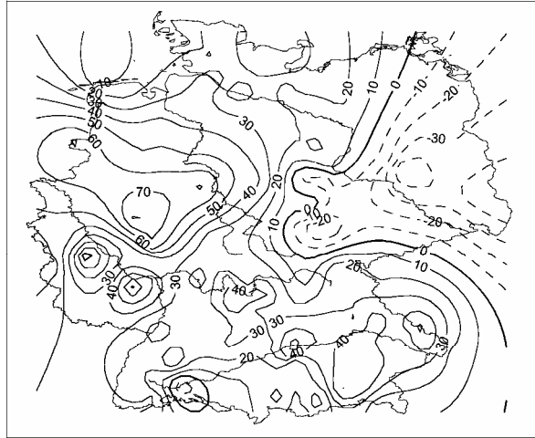
Niederschlag Relativer Trend [% des Mittelwertes] mit signifikanten Gebieten November 1971-2000
