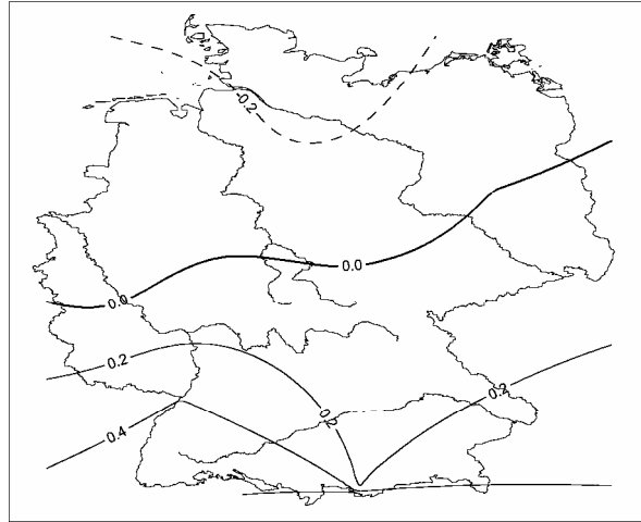
Lufttemperatur Linearer Trend [K] mit signifikanten Gebieten Herbst 1971-2000
