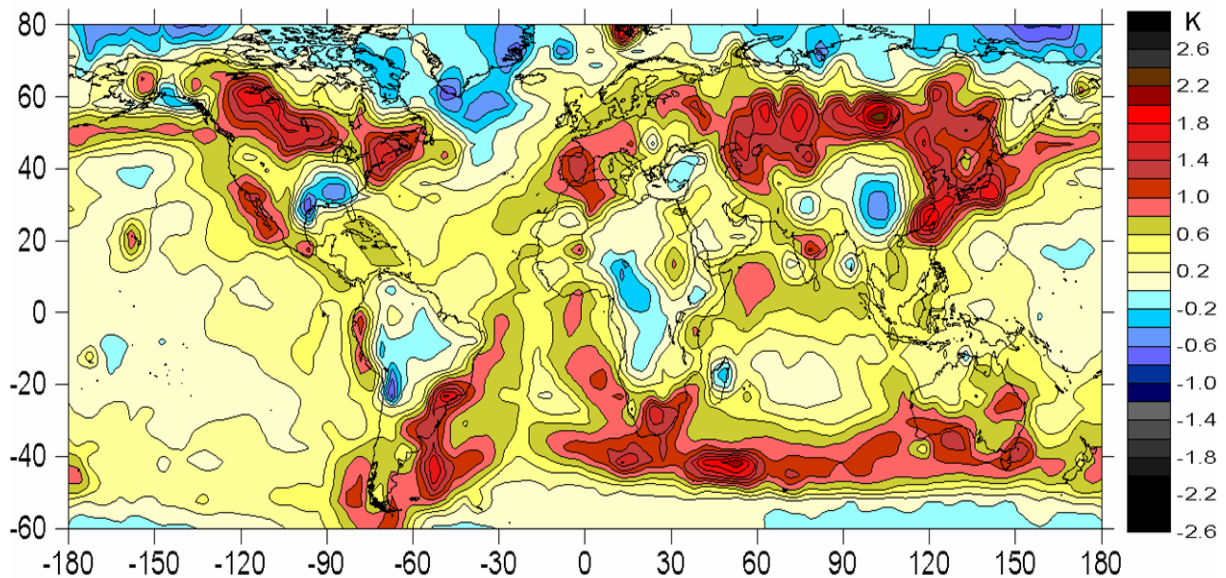
Abb. 2. Globalanalyse der linearen Trends 1901-2000 in °C (K) der bodennahen Lufttemperatur auf der Grundlage eines Gitterrasters 5° x 5° (Datenquelle wie Abb. 1, bearbeitet).
