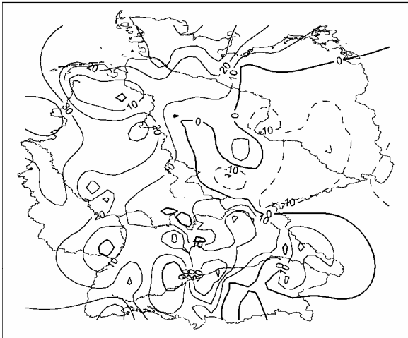
Niederschlag Relativer Trend [% des Mittelwertes] mit signifikanten Gebieten Januar 1931-1960
