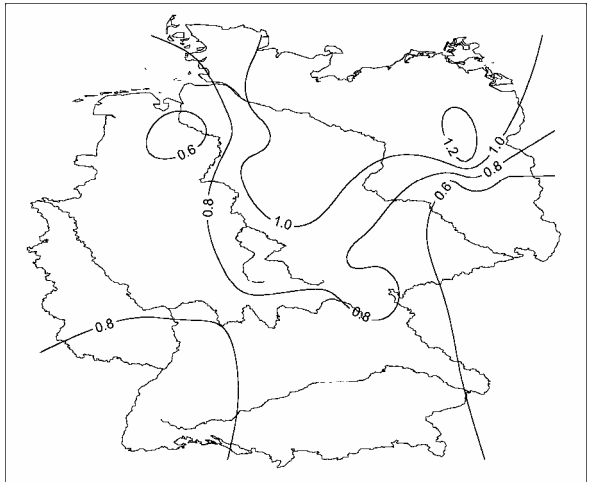
Lufttemperatur Linearer Trend [K] mit signifikanten Gebieten September 1971-2000
