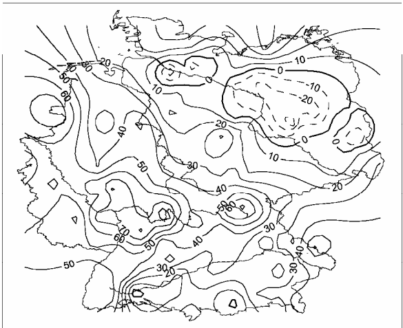
Niederschlag Relativer Trend [% des Mittelwertes] mit signifikanten Gebieten September 1971-2000
