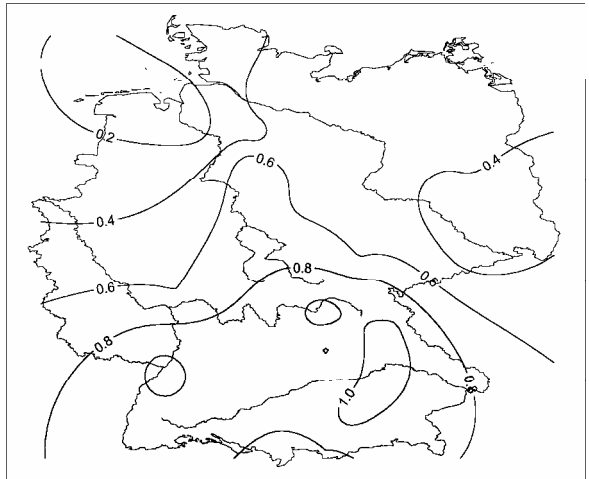
Lufttemperatur Linearer Trend [K] mit signifikanten Gebieten Winter 1931-1960
