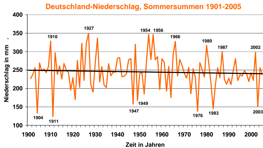
Abb. 14. Sommersummen 1901-2005 des Gebietsniederschlags Deutschland (Datenquelle: DWD) mit linearem Trend.
