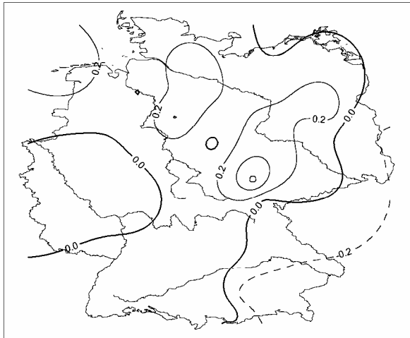
Lufttemperatur Linearer Trend [K] mit signifikanten Gebieten Winter 1901-2000
