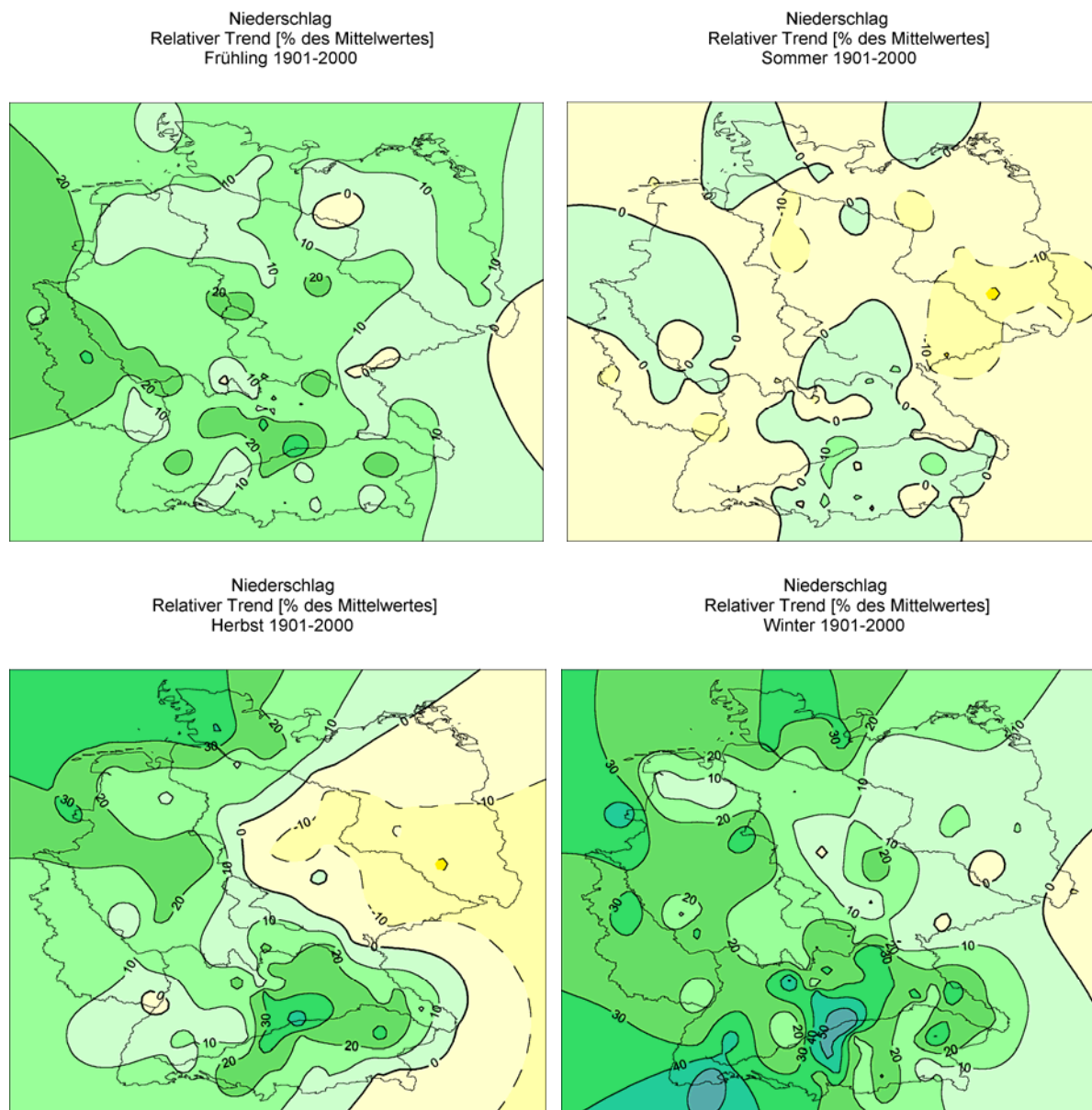
Abb. 18. Karten der linearen Niederschlagstrends 1901-2000 in Prozent, alle vier Jahreszeiten (gelblich Abnahmen, grünlich/bläulich Zunahmen).
