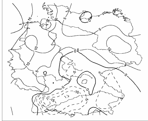
Sonnenscheindauer Linearer Trend [h] mit signifikanten Gebieten Dezember 1971-2000
