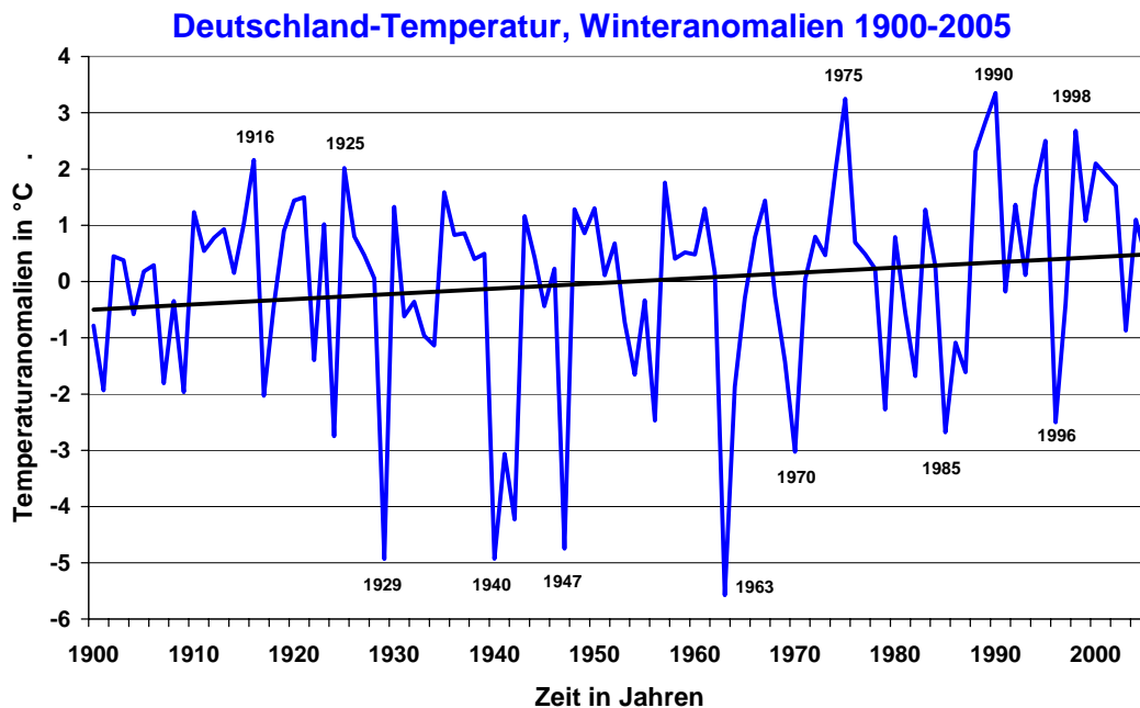
Abb. 12. Ähnlich Abb. 11, jedoch Winter (Dezember des Vorjahrs, Januar, Februar).
