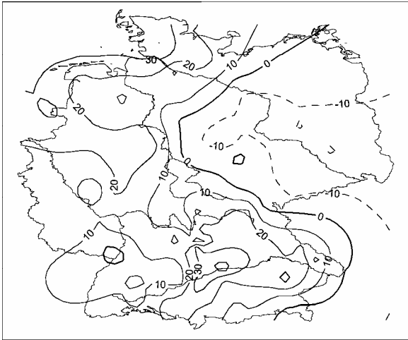
Niederschlag Relativer Trend [% des Mittelwertes] mit signifikanten Gebieten Herbst 1961-1990
