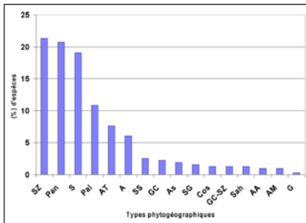
Fig. 6: Spectre des types phytogéographiques du park urban Bangr-Wéogo
