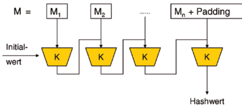
Abbildung 3: Allgemeine Arbeitsweise von Hashfunktionen (nach C. Eckert 17 )
