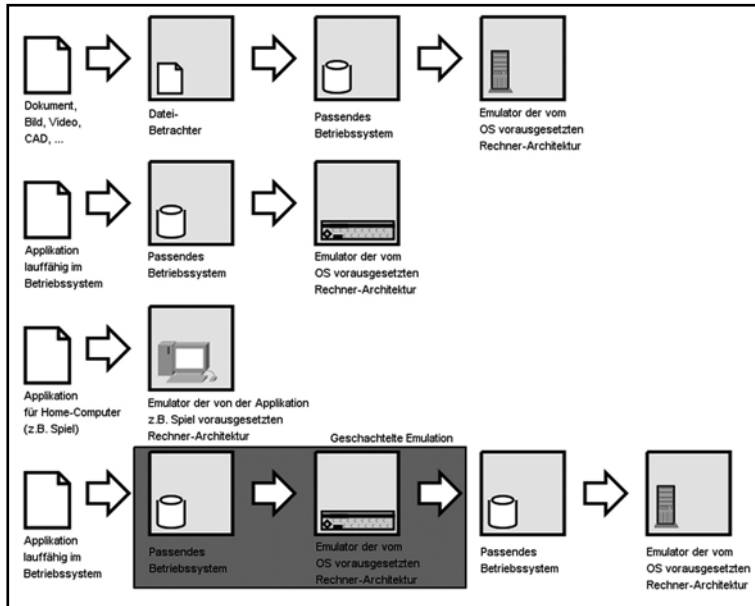
Abbildung 4: Die Länge eines View-Path hängt sowohl vom Typ des Objekts als auch von der eingesetzten Archivierungsstrategie ab.
