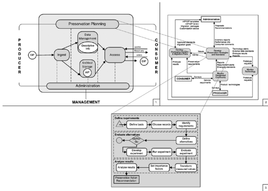
Abbildung 1: OAIS-Modell < Funktionale Entität „Preservation Planning“ < Planungs-Workflow
