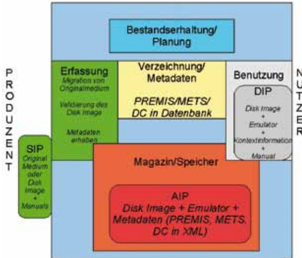
Abbildung 1: OAIS-Funktionsmodell
