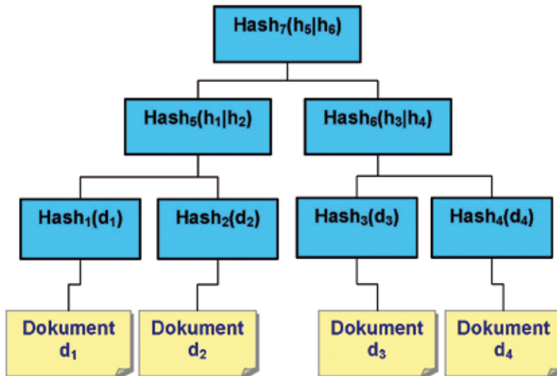
Abbildung 4: Binärer Merkle-Hashbaum.
