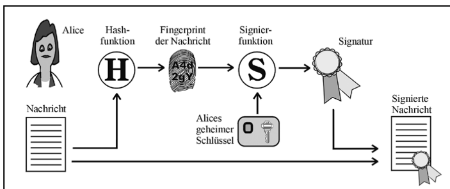
Abbildung 5: Digitale Signatur
